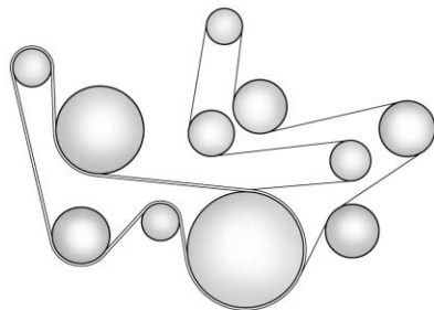
Motor 6.2L LT4
