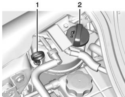
1. Varilla de medición del aceite del motor
