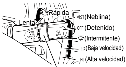
Anillo intermitente
