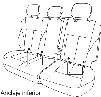
Anclaje inferior del lado trasero izquierdo
