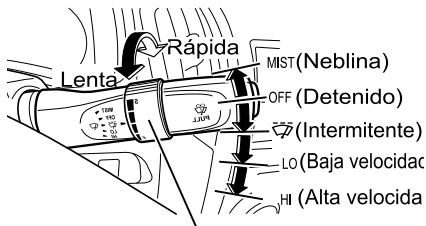
Anillo intermitente
