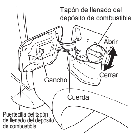
Dispositivo de apertura de la tapa del combustible
