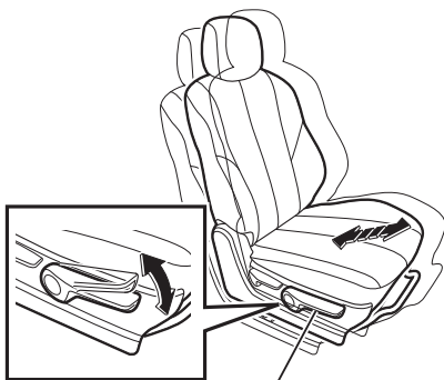
Palanca de ajuste de la altura
