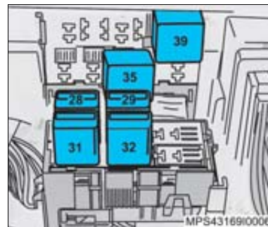
Central eléctrica secundaria (debajo del asiento del conductor)
