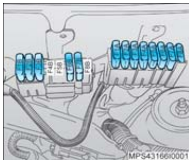
Caja de maxifusibles en el cofre
