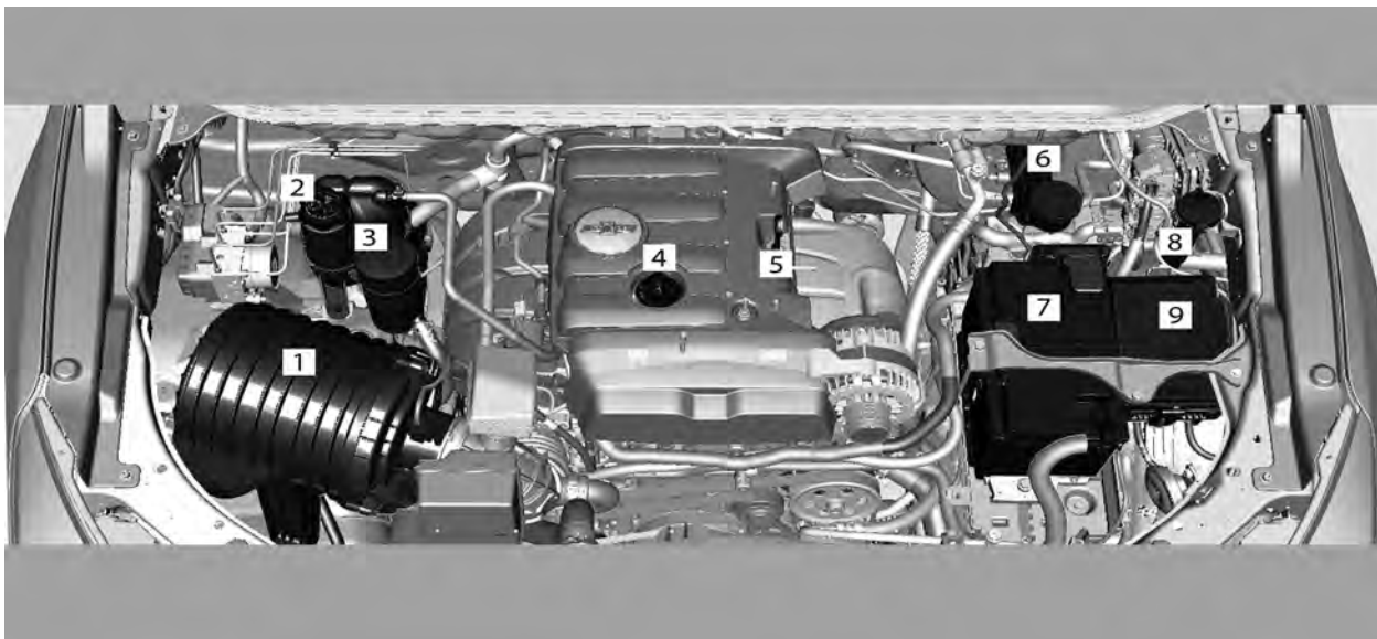
Motor de nafta / flex, 2.5L ECOTEC
