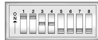
Ejemplo de ocho interruptores DIP con tres posiciones
