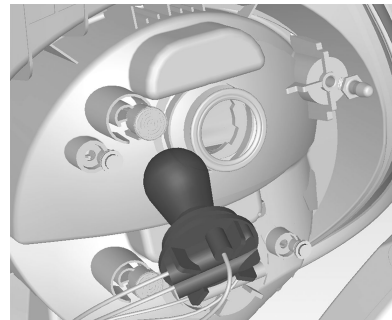
4. Gire el portalámparas en sentido antihorario.
