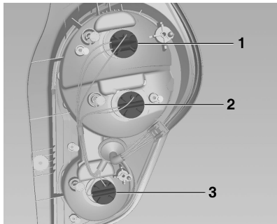
3. Luz trasera / luz de freno (1) Intermitente (2) Luz de marcha atrás (lado del acompañante) / Piloto antiniebla (lado del conductor) (3)
