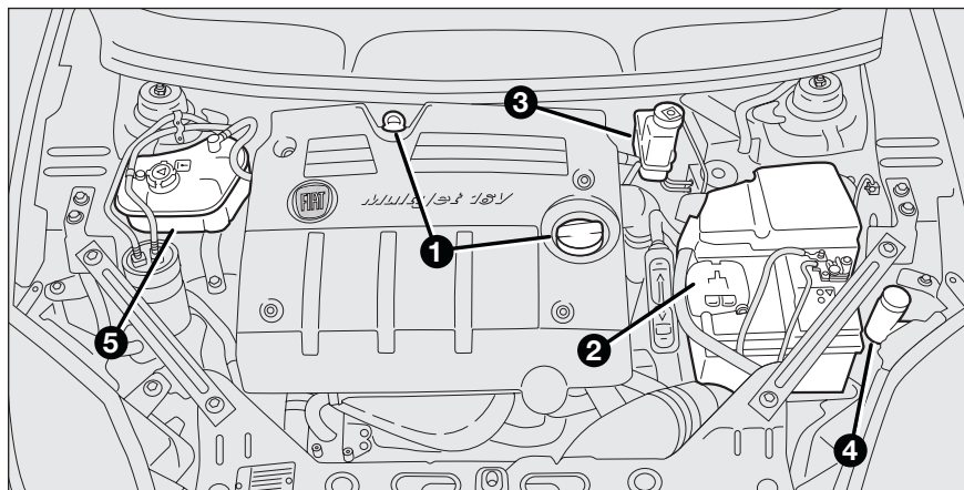
fig. 5 - versión 1.9 Multijet 16V
