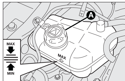
fig. 12 - versiones 1.4 T-JET, 1.6 Multijet, 1.9 Multijet
