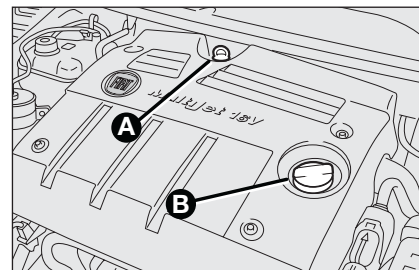
fig. 10 - versión 1.9 Multijet 16V
