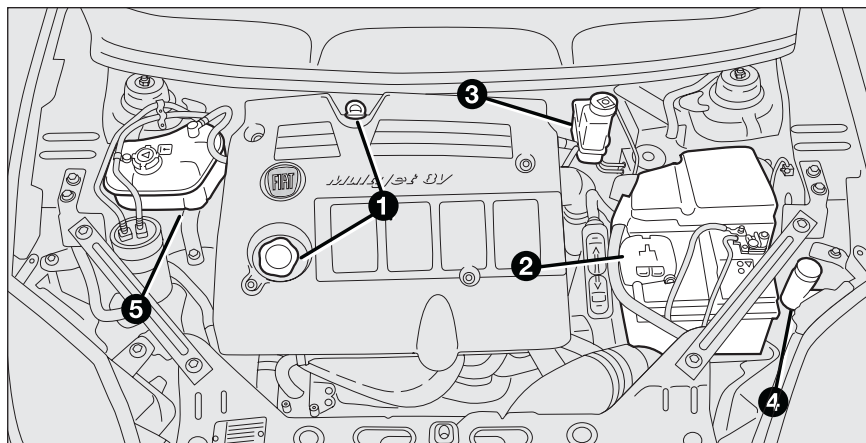
fig. 4 - versión I.9 Multijet 8v
