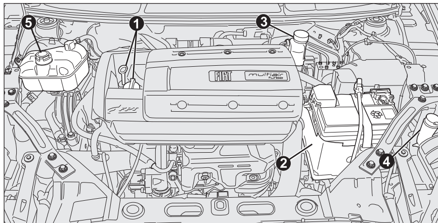
fig. 2a - versión 1.4 Turbo Multi Air
