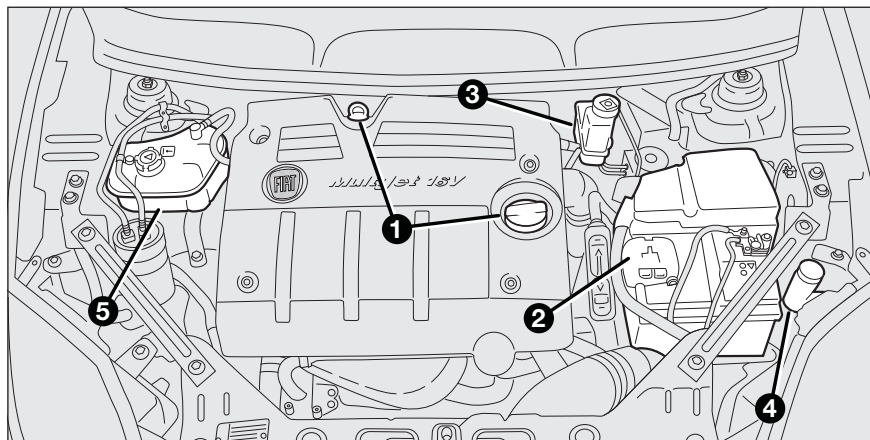
fig. 5 - versión 1.9 Multijet 16V (para las versiones/paises donde esté previsto)
