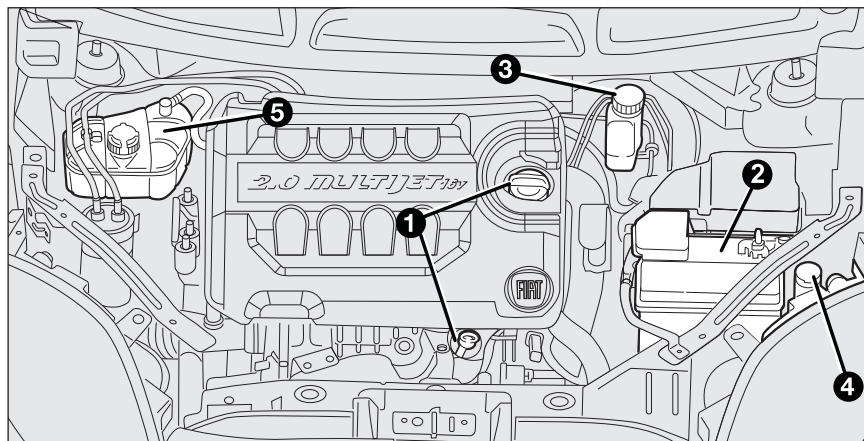
fig. 5a - versión 2.0 Multijet
