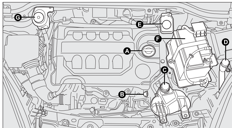
fig. 183 - Versiones 1.6 Multijet
