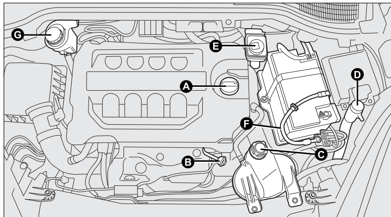
fig. 184 - Versiones 2.0 Multijet
