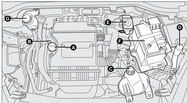
fig. 180 - Versiones 1.4
