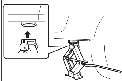
Rueda trasera
