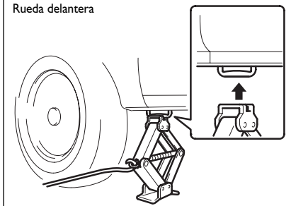
Rueda delantera
