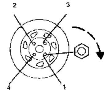
Secuencia de apriete de las tuercas de rueda
