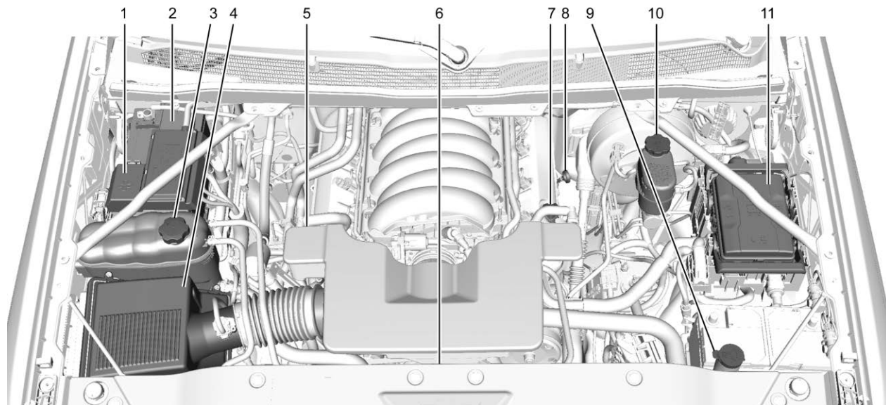
Motor 6.2L V8
