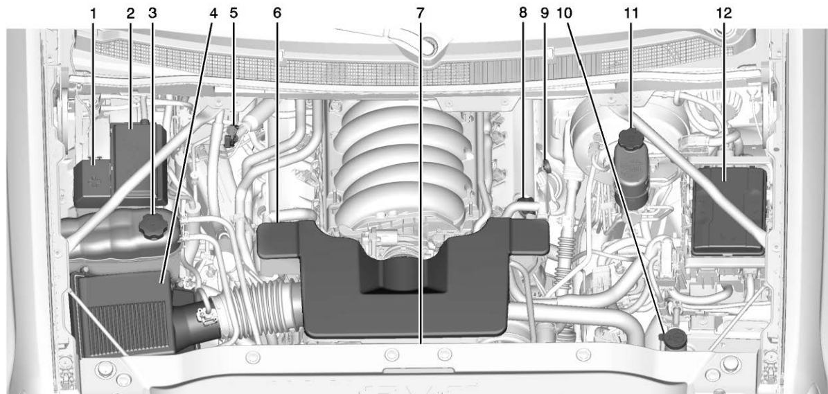
Motor 5.3L V8
