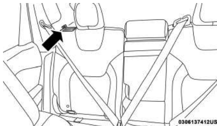
Palanca de liberación del asiento fijo trasero
