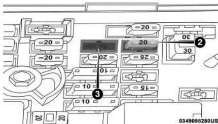
Ubicaciones de fusibles de tomas de corriente del área de carga trasera
