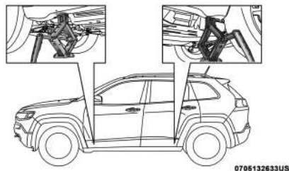
Puntos de apoyo del gato
