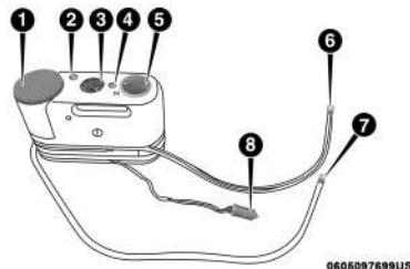
Componentes del equipo de servicio para neumáticos
