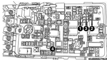
Ubicación de los fusibles de la toma de corriente
