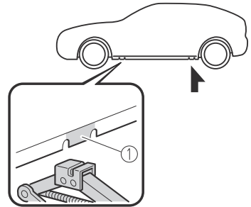
1. Posición de instalación del gato
