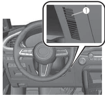
1. Sensor de temperatura interior
