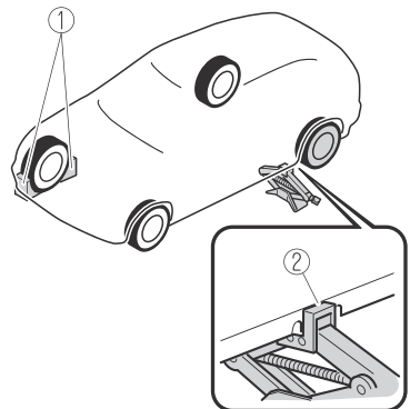
1. Bloques para neumáticos 2. Posición de instalación del gato
