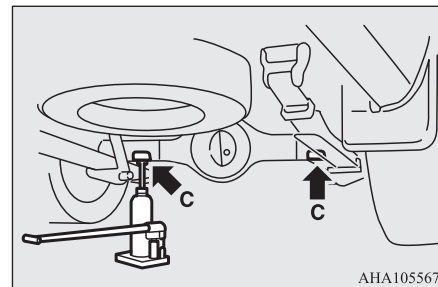
C- Punto de elevación con gato trasero
