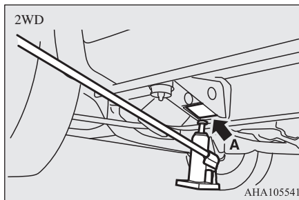
A- Punto de elevación con gato delantero (vehículos de 2WD)
