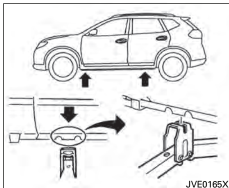
Punto de elevación
