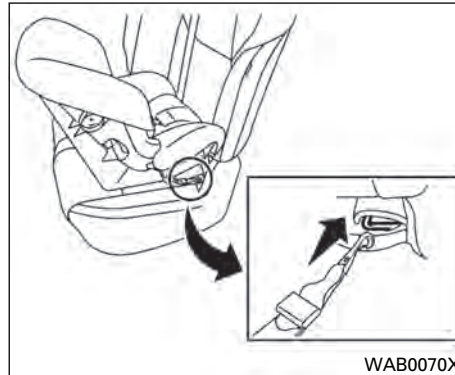
Montado en cincha orientado hacia atrás: paso 2
