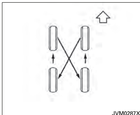
Los neumáticos no tienen flechas que muestran la dirección de rotación
