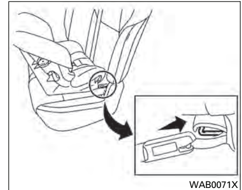
Montaje rígido orientado hacia atrás: paso 2
