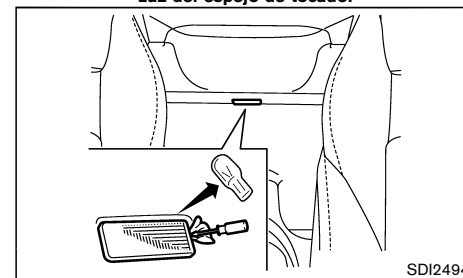
Luz de cortesía del área para carga - Roadster
