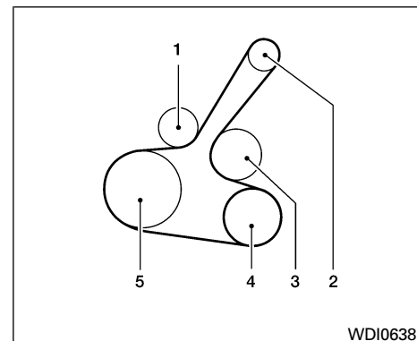
Modelo MR20DE
