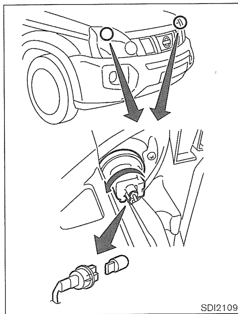
Luz de señal direccional delantera
