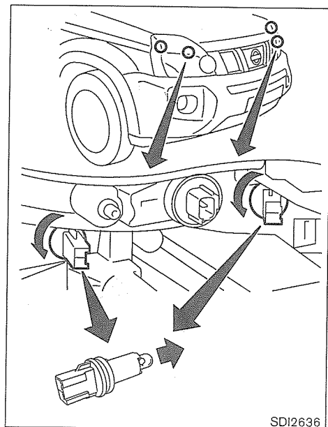
Luz de despejo tipo B
