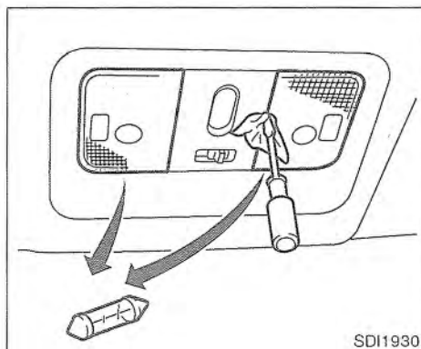
Luz de mapas delantera
