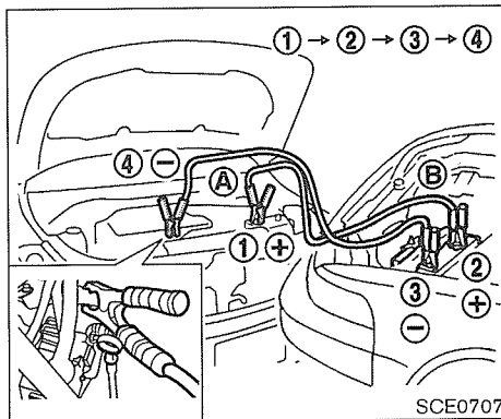
Modelo con motor QR25
