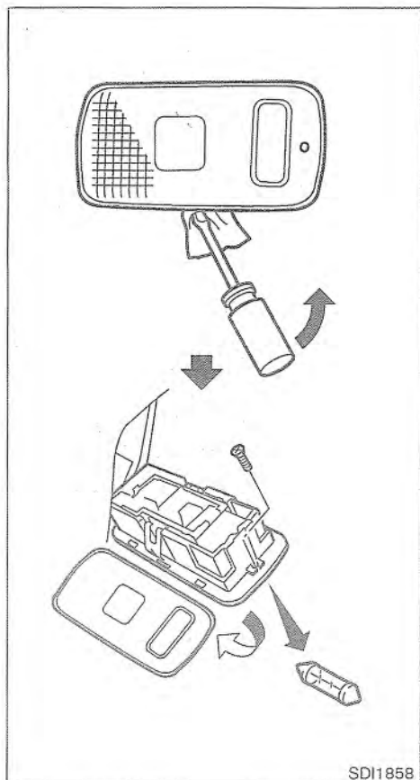
Luz personal trasera/luz de compartimiento para equipajes (lado de la carrocería)
