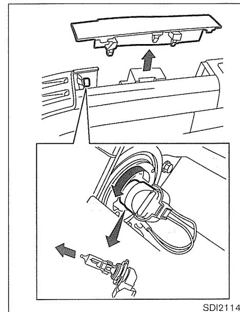
Luz de conducción (si está equipada)
