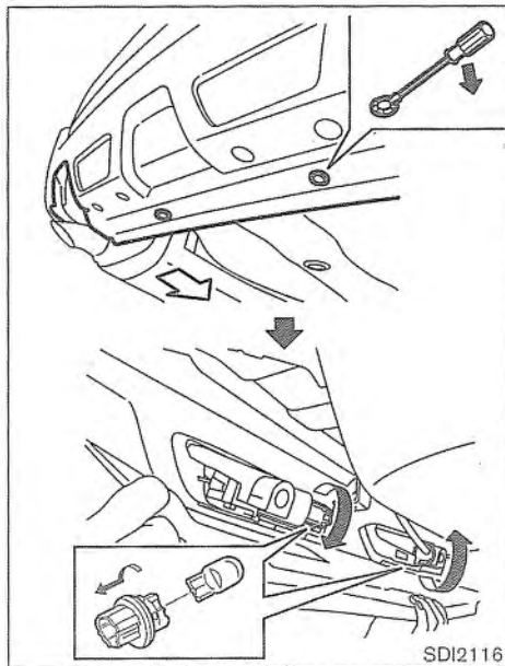
Luz antiniebla trasera y de marcha atrás
