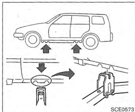
Puntos de elevación
