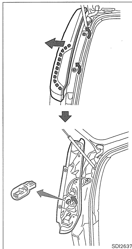
Luz combinada trasera tipo B
