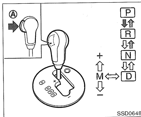
Modelo con volante a la izquierda (LHD)
