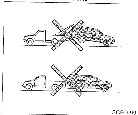
Modelo 2WD (modelos AT y CVT)
