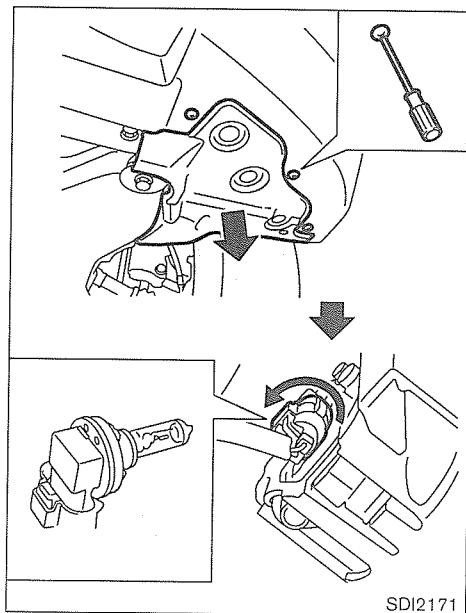
Luz antiniebla delantera (si está equipada)
