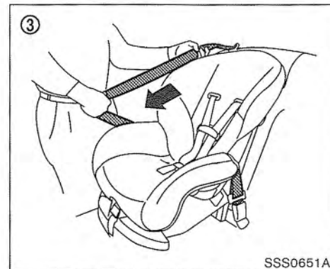
Orientado hacia adelante: Paso 4
