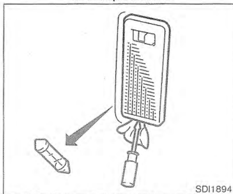
Luz de compartimiento para equipajes (lado de la puerta)
