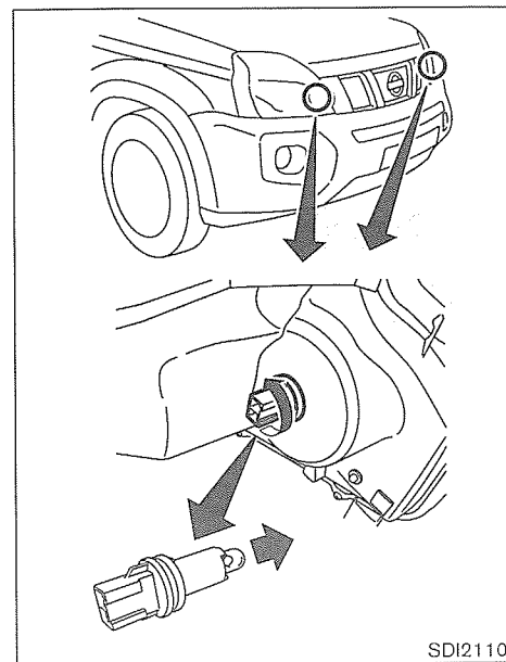
Luz de despejo tipo A
