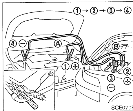
Modelo con motor MR20
