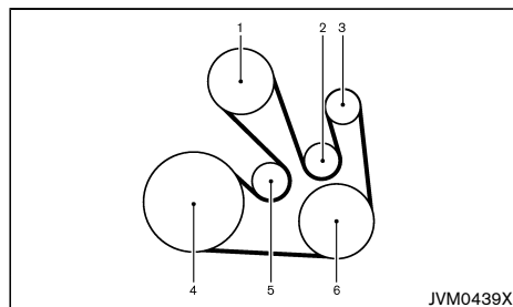
Motor R9M
