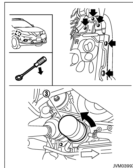
Motor QR25DE
