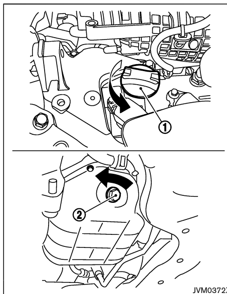
Motor QR25DE
