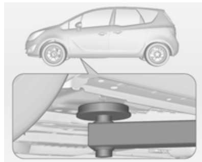
Posición del brazo delantero de la plataforma elevadora en los bajos.
