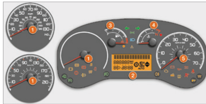
Cuadro de a bordo con pantalla de nivel 2
