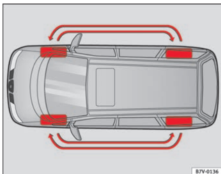
Fig. 149 Esquema para el cambio de ruedas
