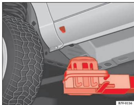
Fig. 174 Punto de apoyo en la parte delantera izquierda para elevar el vehículo con la plataforma
