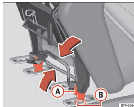
Fig. 93 Montaje del asiento: estribos y pernos
