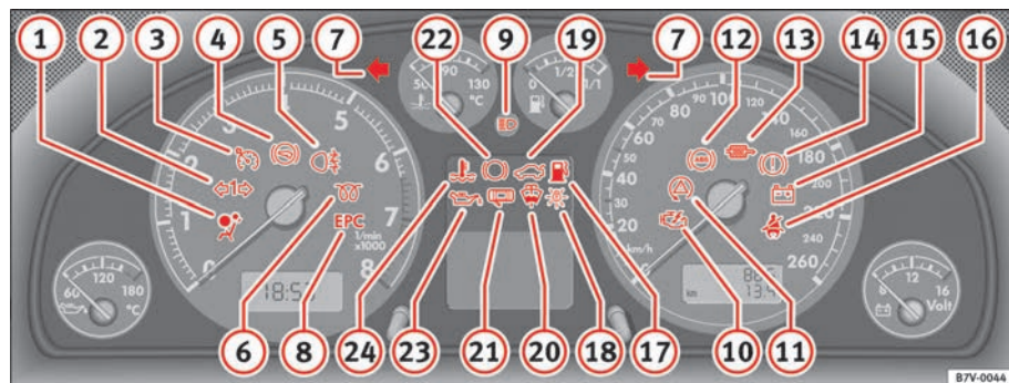
Fig. 48 Testigos de control y de advertencia del cuadro de instrumentos. Algunos de estos testigos pertenecen sólo a determinadas versiones del modelo o forman parte de equipamientos opcionales.
