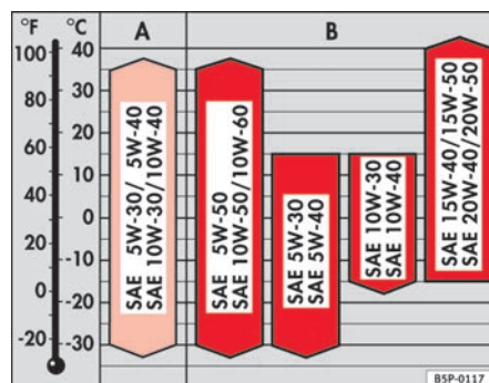
Fig. 139 Tipos de aceite de acuerdo a la temperatura
