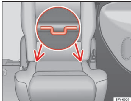
Fig. 33 Argollas de sujeción para los asientos para niños con el sistema ISOFIX en el armazón de los asientos de la segunda fila
