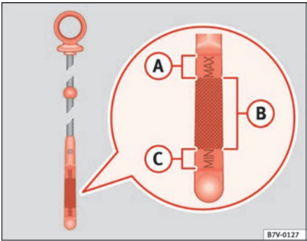
Fig. 140 Varilla de medición de aceite
