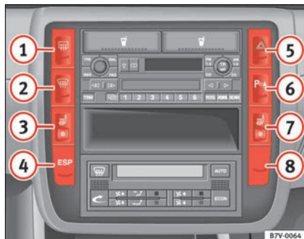
Fig. 77 Consola central: tecla de la luneta térmica
