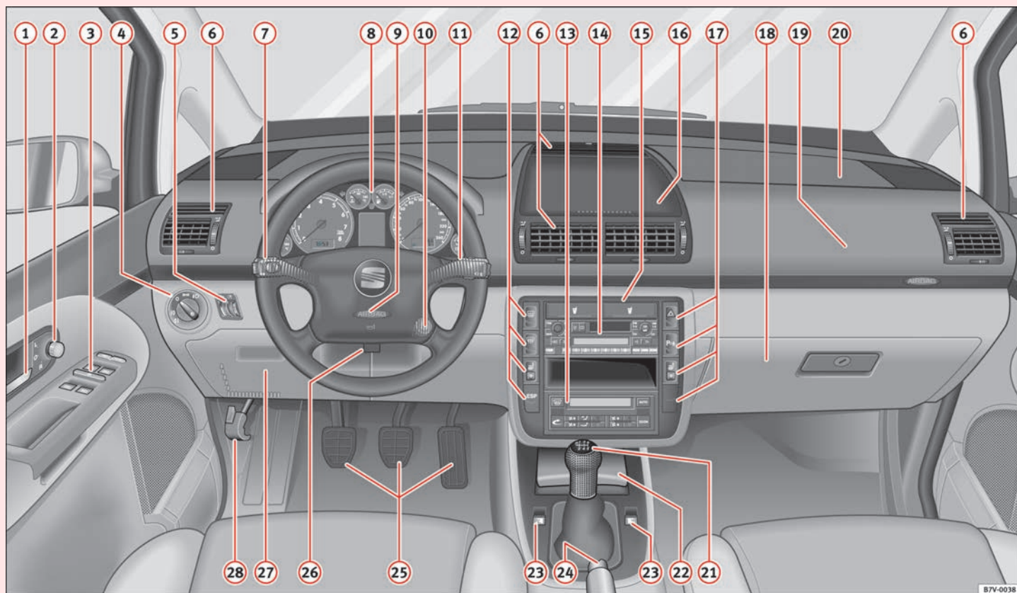
Fig. 43 Tablero de instrumentos
