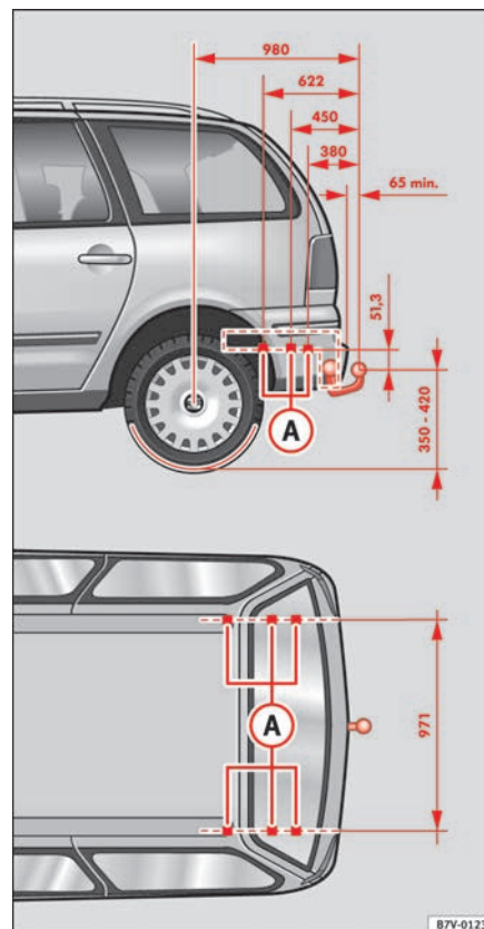
Fig. 135 Puntos de fijación del enganche de remolque
