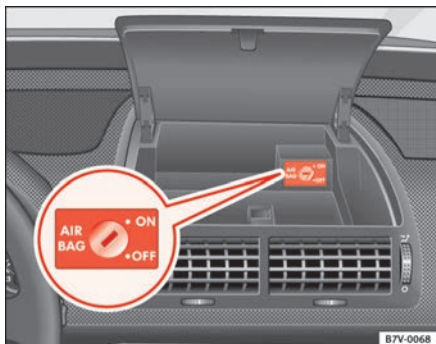
Fig. 28 Interior del compartimento del centro del tablero de instrumentos: interruptor de llave para desactivar los airbags del acompañante
