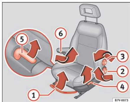
Fig. 86 Mandos del asiento delantero izquierdo
