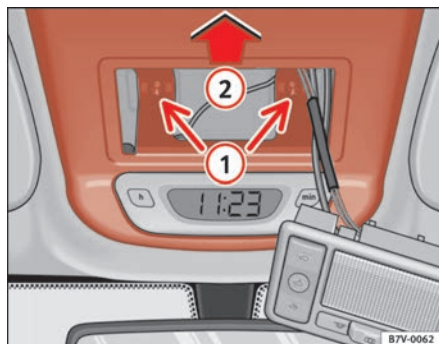
Fig. 68 Accionamiento de emergencia
