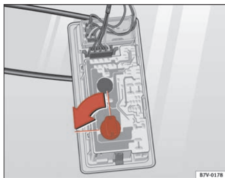
Fig. 170 Luz de lectura
