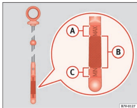
Fig. 141 Varilla de medición de aceite
