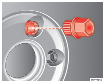
Fig. 159 Cambio de rueda: tornillo de rueda antirrobo y adaptador
