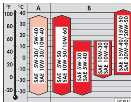
Fig. 140 Tipos de aceite de acuerdo a la temperatura
