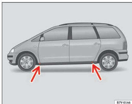
Fig. 160 Puntos de apoyo del gato
