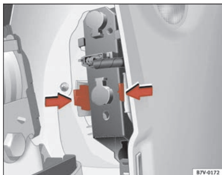
Fig. 165 Luces en la carrocería
