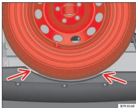
Fig. 153 Rebaje para la rueda de repuesto en el paragolpes
