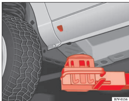
Fig. 175 Punto de apoyo en la parte delantera izquierda para elevar el vehículo con la plataforma
