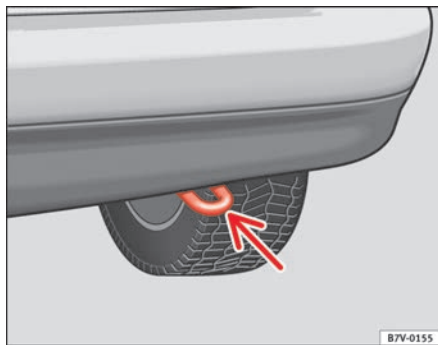
Fig. 174 Argolla de remolque trasera
