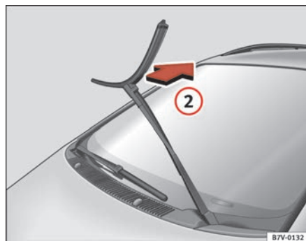
Fig. 146 Desmontaje de los limpiaparabrisas delanteros
