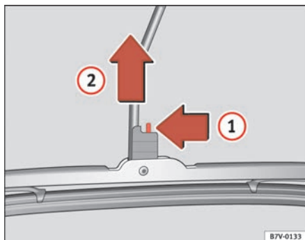
Fig. 147 Cambio del limpialuneta
