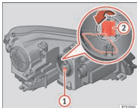
Fig. 203 Portalámparas del intermitente ① y luz para curvas ②.
