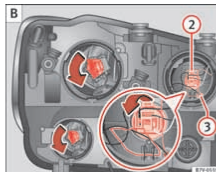
Fig. 201 Faro izquierdo
