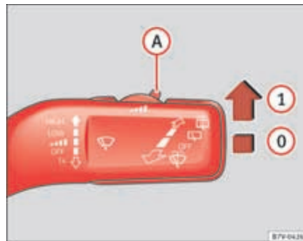
Fig. 69 Palanca del limpiaparabrisas: ajustar el sensor de lluvia (A).
