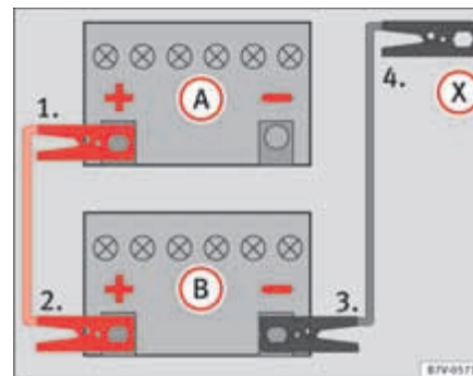
Fig. 213 Esquema de conexión de los cables de emergencia cuando un vehículo sin sistema Start-Stop suministra la corriente: batería descargada (A) y batería que suministra la corriente (B).
