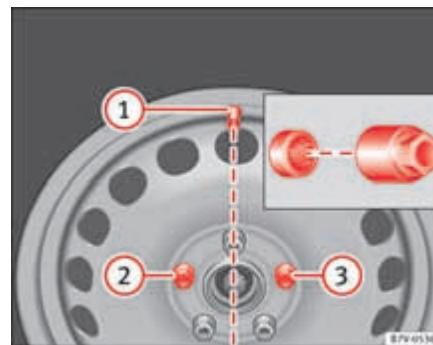
Fig. 179 Cambio de rueda: Válvula del neumático ① y ubicación del tornillo antirrobo de la rueda ② o ③.
