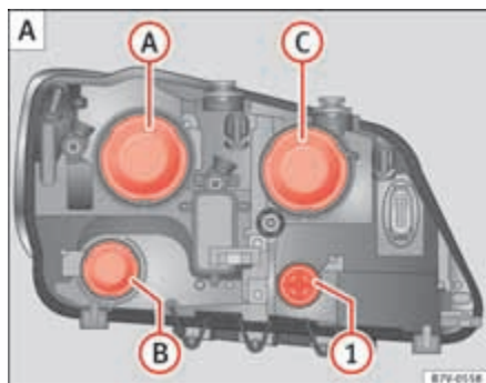
Fig. 200 En el vano motor: Revestimientos en el faro izquierdo. A) luces de cruce, B) luz diurna y C) luz de carretera y luz de posición.
