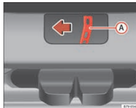
Fig. 189 Desde el maletero: Desbloqueo de emergencia del portón trasero.
