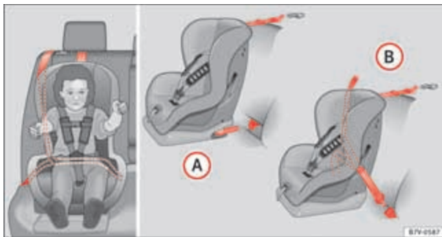
Fig. 26 En los asientos traseros: la ilustración (A) muestra la fijación básica del sistema de retención para niños con las anillas de sujeción inferiores y el cinturón de sujeción superior. La ilustración (B) muestra la fijación del sistema de retención para niños con el cinturón de seguridad del vehículo.
