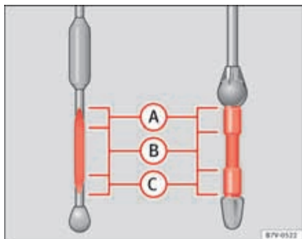
Fig. 165 Varilla de medición con marcas para el nivel del aceite.
