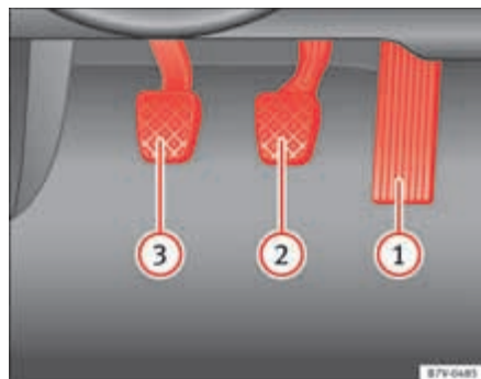
Fig. 127 Pedales en vehículos con cambio manual: ① acelerador; ② freno; ③ embrague.
