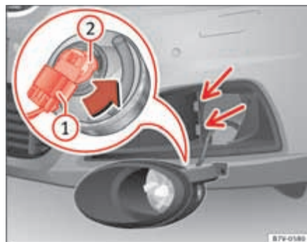
Fig. 205 Cambio de las lámparas de los faros.
