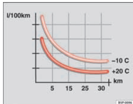
Fig. 152 Consumo de combustible (l/100 km) a diferente temperatura ambiental.
