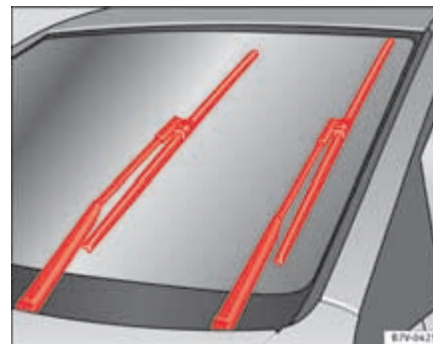
Fig. 68 Limpiaparabrisas en posición de servicio. ►
