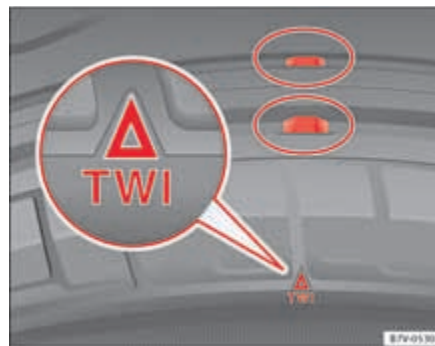
Fig. 174 Perfil del neumático: indicadores de desgaste.
