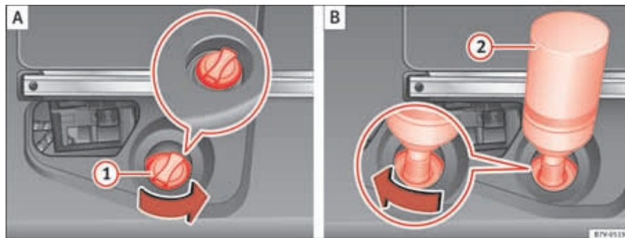
Fig. 162 Depósito de AdBlue con cierre de la boca de llenado y botella para reponer.
