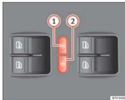
Fig. 52 En la puerta del conductor: teclas del seguro eléctrico para niños.
