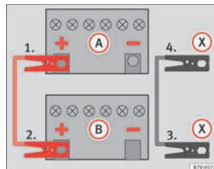
Fig. 214 Esquema de conexión de los cables de emergencia cuando un vehículo con sistema Start-Stop suministra la corriente: batería descargada (A) y batería que suministra la corriente (B).
