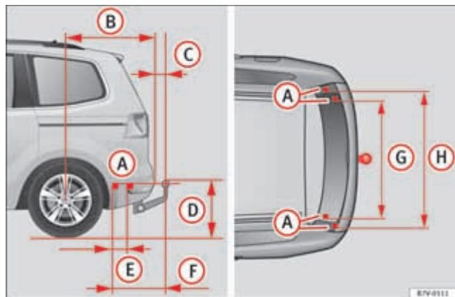
Fig. 154 Cotas y puntos de fijación para instalar posteriormente un enganche para remolque.
