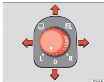
Fig. 73 En la puerta del conductor; mando de los retrovisores exteriores.
