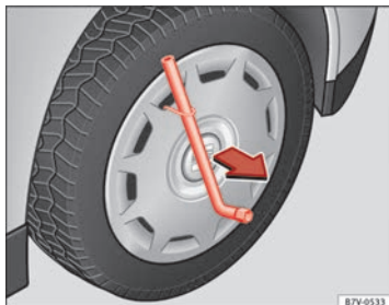
Fig. 181 Desmontar el tapacubos integral.
