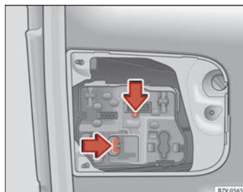
Fig. 212 En el portón trasero: Retirar el portalámparas.
