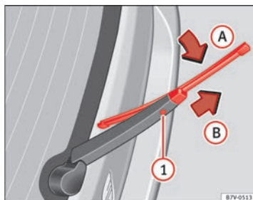
Fig. 161 Cambio de la escobilla de la luneta.
