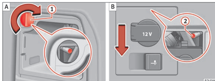
Fig. 213 En el lateral del maletero: Desmontar las luces posteriores izquierda y derecha. ① retirar el capuchón; ② tornillo de fijación.
