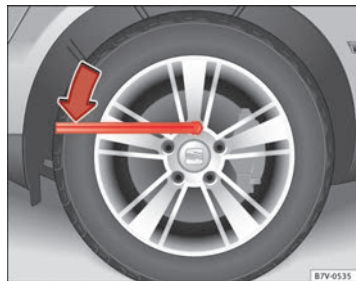
Fig. 183 Cambio de rueda: afloje los tornillos de la rueda.
