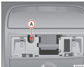
Fig. 196 Tornillo Allen para cerrar el techo corredizo panorámico.
