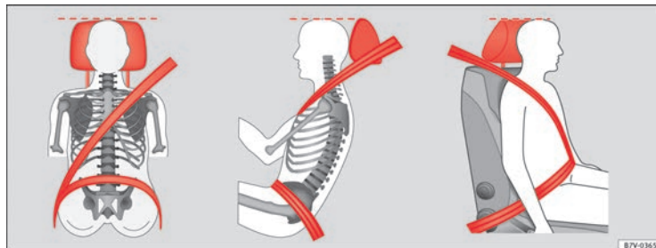
Fig. 13 Banda del cinturón y apoyacabezas ajustados correctamente.
