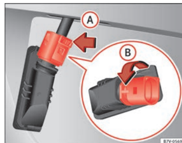
Fig. 216 Luz de la matrícula: Desmontar el portalámparas.
