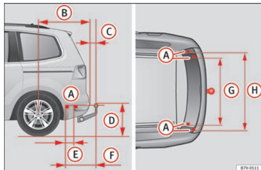
Fig. 159 Cotas y puntos de fijación para instalar posteriormente un enganche para remolque.
