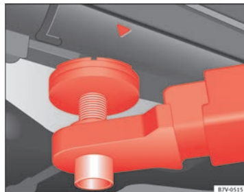
Fig. 163. Puntos de apoyo traseros para elevar el vehículo con la plataforma elevadora o con el gato.
