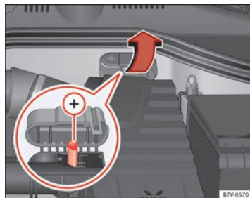
Fig. 217 En el vano motor: polo positivo de ayuda de arranque (+).
