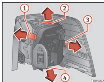
Fig. 214 Luz trasera en la carrocería: Desmontar el portalámparas. ① a ④: lengüetas de bloqueo.
