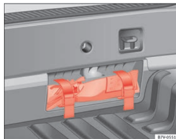
Fig. 199 En el maletero, visto desde el interior del vehículo: Herramientas de a bordo en una cavidad situada en la zona del portacierres.
