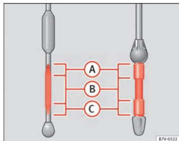
Fig. 170 Varilla de medición con marcas para el nivel del aceite.
