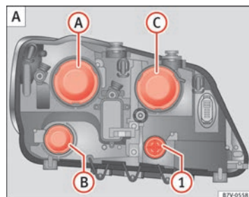
Fig. 205 En el vano motor: Revestimientos en el faro izquierdo. (A) luces de cruce, (B) luz diurna y (C) luz de carretera y luz de posición.
