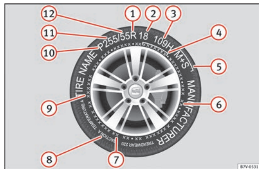
Fig. 180 Inscripción universal en los neumáticos.
