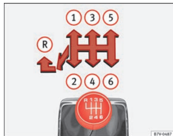
Fig. 131 Esquema de un cambio manual de 6 marchas.
