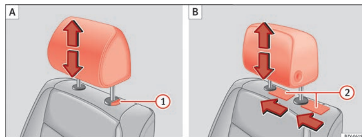
Fig. 86 A: Montaje de los apoyacabezas sin posibilidad de regulación en dirección longitudinal, B: Montaje de los apoyacabezas con posibilidad de regulación en dirección longitudinal.
