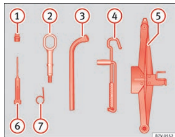
Fig. 200 Componentes del juego de herramientas de a bordo.
