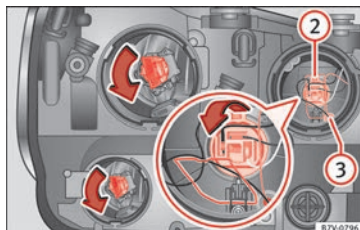
Fig. 212 Faro izquierdo.
