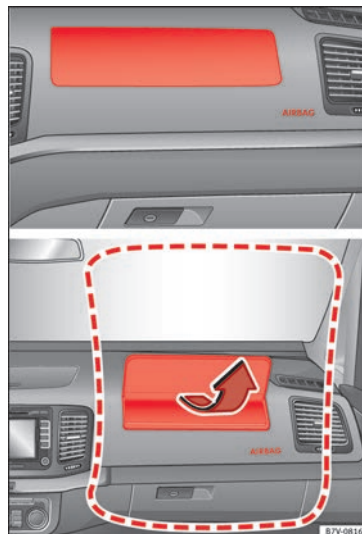
Fig. 14 Ubicación y campo de acción del airbag frontal del acompañante.
