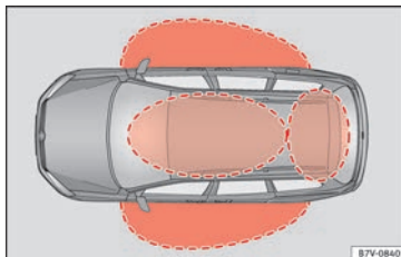
Fig. 46 Sistema de cierre y arranque sin llave Keyless Access: zonas próximas.
