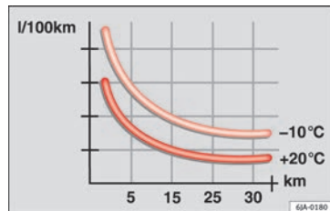
Fig. 133 Consumo de combustible (l/100 km) a diferente temperatura ambiental.
