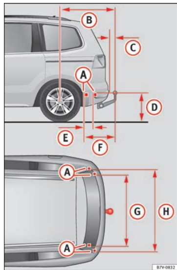
Fig. 155 Cotas y puntos de fijación para instalar posteriormente un enganche para remolque.
