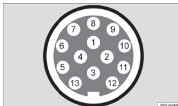
Fig. 154 Representación esquemática: asignación de los pines de la toma de corriente del remolque.
