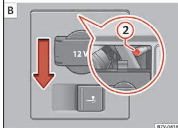
Fig. 219 En el lateral del maletero: desmontar las luces posteriores izquierda y derecha. ① retirar el capuchón; ② tornillo de fijación.
