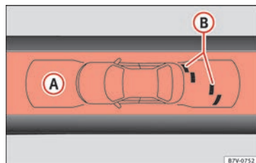
Fig. 140 Indicación del OPS en pantalla: (A) se ha detectado un obstáculo en el segmento; (B) zona registrada delante del vehículo.
