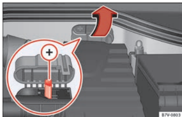
Fig. 191 En el vano motor: polo positivo de ayuda de arranque (+).
