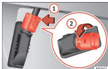
Fig. 222 Luz de la matrícula: Desmontar el portalámparas.
