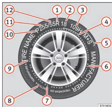
Fig. 177 Inscripción universal en los neumáticos.
