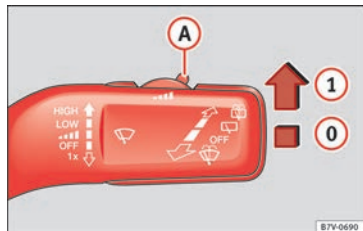
Fig. 67 Palanca del limpiaparabrisas: ajustar el sensor de lluvia ❶.
