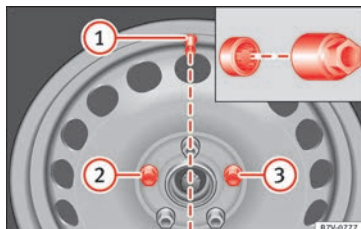
Fig. 186 Cambio de rueda: válvula del neumático ① y ubicación del tornillo antirrobo de la rueda ② o ③.
