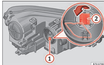
Fig. 214 Portalámparas del intermitente ① y luz para curvas ②.
