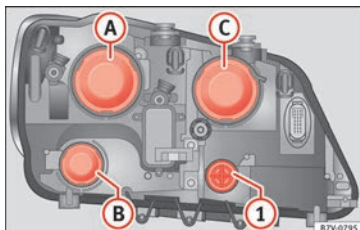
Fig. 211 En el vano motor: revestimientos en el faro izquierdo. A luces de cruce, B luz diurna y C luz de carretera y luz de posición.
