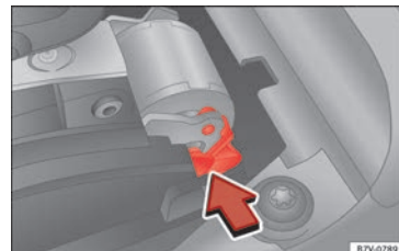
Fig. 204 Desbloqueo de emergencia del bloqueo de la palanca selectora.
