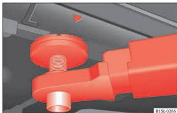
Fig. 234 Puntos de apoyo traseros para elevar el vehículo con la plataforma elevadora o con el gato.
