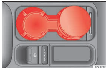
Fig. 192 Consola central delantera: cenicero cerrado.
