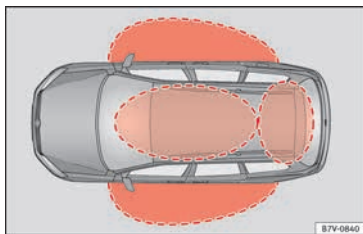
Fig. 132 Sistema de cierre y arranque sin llave Keyless Access: zonas próximas.
