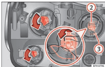
Fig. 107 Faro izquierdo.
