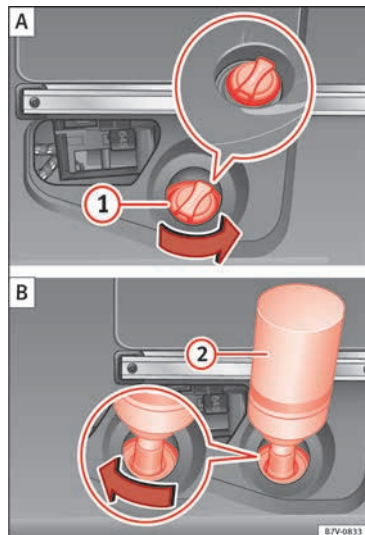
Fig. 238 Depósito de AdBlue con cierre de la boca de llenado y botella para reponer.
