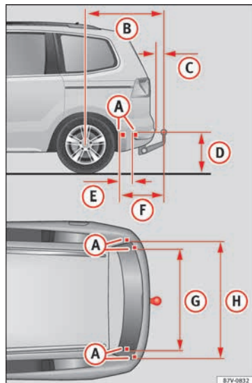
Fig. 232 Cotas y puntos de fijación para instalar posteriormente un enganche para remolque.
