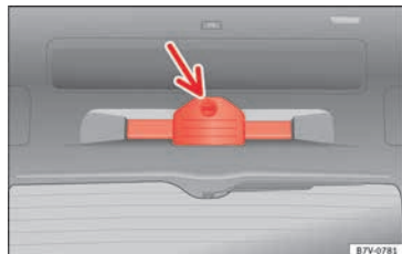
Fig. 99 En el portón trasero: Soporte de triángulo de preseñalización.
