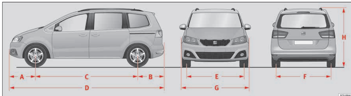
Fig. 256 Dimensiones
