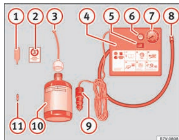
Fig. 103 Representación estándar: contenido del kit antipinchazos.
