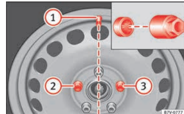
Fig. 69 Cambio de rueda: válvula del neumático ① y ubicación del tornillo antirrobo de la rueda ② o ③.
