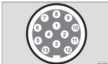
Fig. 231 Representación esquemática: asignación de los pines de la toma de corriente del remolque.
