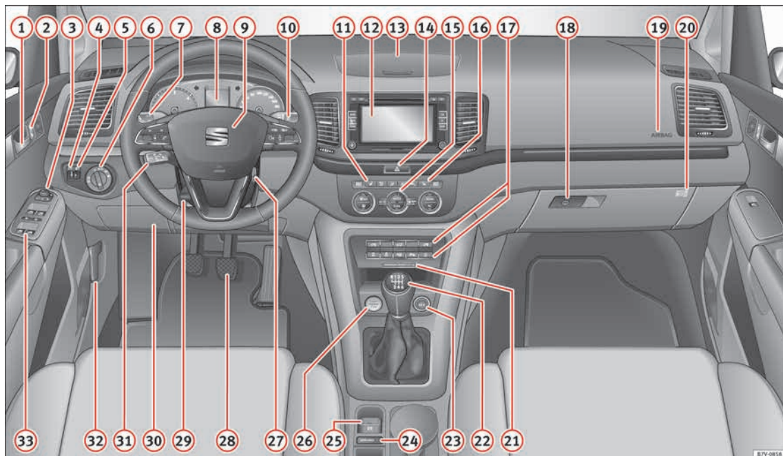
Fig. 118 Tablero de instrumentos.
