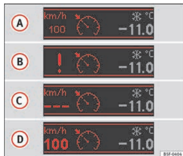
Fig. 219 Pantalla del cuadro de instrumentos: indicaciones de estado del GRA.
