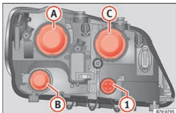
Fig. 106 En el vano motor: revestimientos en el faro izquierdo. A luces de cruce, B luz diurna y C luz de carretera y luz de posición.
