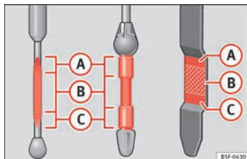
Fig. 242 Varilla de medición con marcas para el nivel del aceite.
