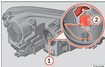
Fig. 109 Portalámparas del intermitente (1) y luz para curvas (2).
