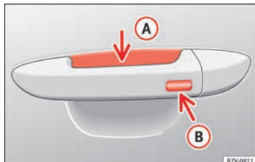
Fig. 133 Sistema de cierre y arranque sin llave Keyless Access: superficie sensora (A) de desbloqueo en la parte interior de la manija de la puerta y superficie sensora (B) de bloqueo en la parte exterior de la manija.
