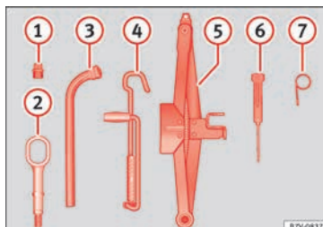
Fig. 101 Componentes del juego de herramientas de a bordo.
