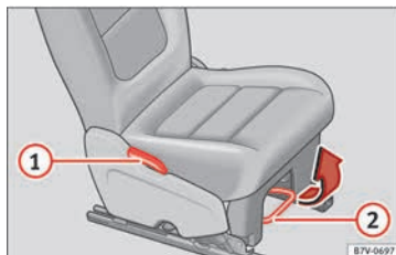
Fig. 150 Ajustar los asientos traseros.
