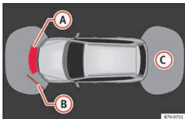
Fig. 211 Indicación del OPS en pantalla: (A) se ha detectado un obstáculo en la zona de colisión; (B) se ha detectado un obstáculo en el segmento; (C) zona registrada detrás del vehículo.
