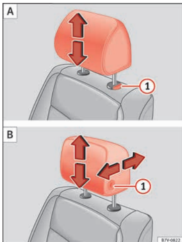
Fig. 151 A: Ajuste de los apoyacabezas sin posibilidad de regulación en dirección longitudinal; B: Ajuste de los apoyacabezas con posibilidad de regulación en dirección longitudinal.
