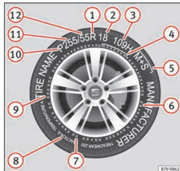
Fig. 254 Inscripción universal en los neumáticos.
