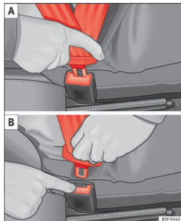
Fig. 88 Inserte la lengüeta del cinturón de seguridad en el cierre.
