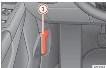
Fig. 239 En la zona reposapiés, en el lado del conductor: Palanca para el desbloqueo del capó del motor.
