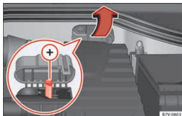
Fig. 75 En el vano motor: polo positivo de ayuda de arranque (+).
