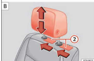
Fig. 153 A: Montaje de los apoyacabezas sin posibilidad de regulación en dirección longitudinal; B: Montaje de los apoyacabezas con posibilidad de regulación en dirección longitudinal.
