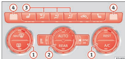
Fig. 53 Detalle de la consola central: Mandos del Climatronic.
