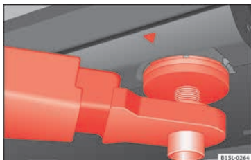
Fig. 233 Puntos de apoyo delanteros para elevar el vehículo con la plataforma elevadora o con el gato.
