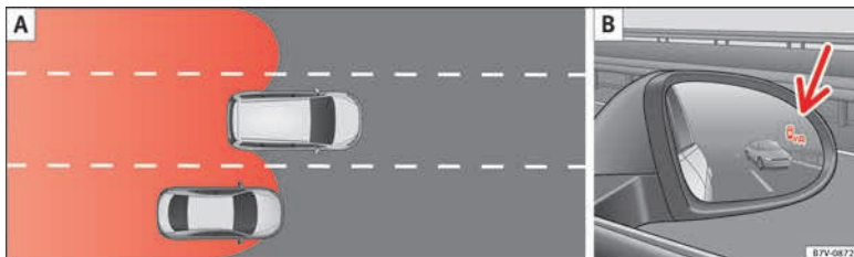
Fig. 224 Representación esquemática: A Situación en un adelantamiento e incorporación posterior al carril derecho. B Indicación del asistente de ángulo muerto en el retrovisor exterior derecho.
