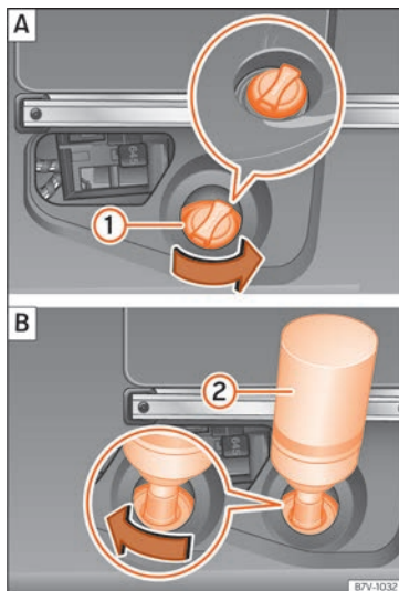
Fig. 285 Depósito de AdBlue con cierre de la boca de llenado y botella para reponer.
