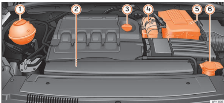
Fig. 288 Figura orientativa de la posición de los elementos.
