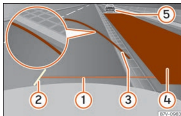
Fig. 278 Pantalla: líneas y superficies de orientación del espacio detrás del vehículo.
