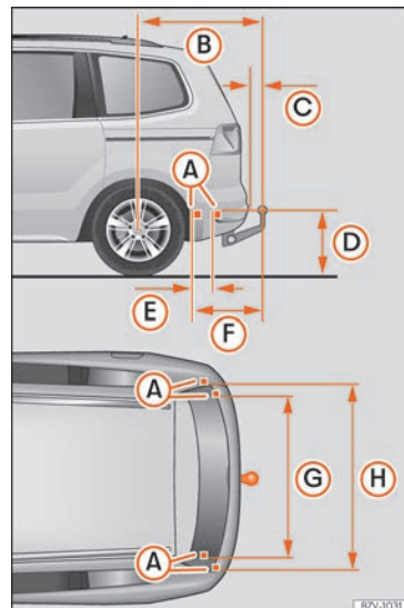
Fig. 281 Cotas y puntos de fijación para el montaje posterior de un dispositivo de remolque.
