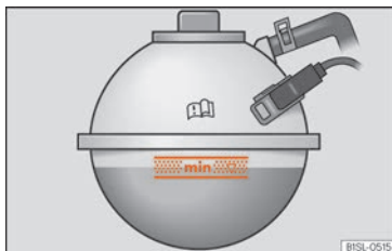
Fig. 291 En el vano motor: marca en el depósito de expansión del líquido refrigerante.
