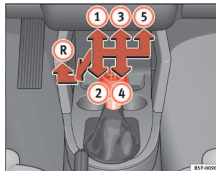
Fig. 132 Detalle de la consola central: esquema de un cambio manual de 5 marchas
