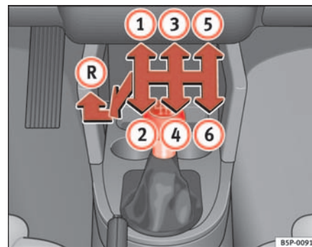
Fig. 133 Detalle de la consola central: esquema de un cambio manual de 6 marchas
