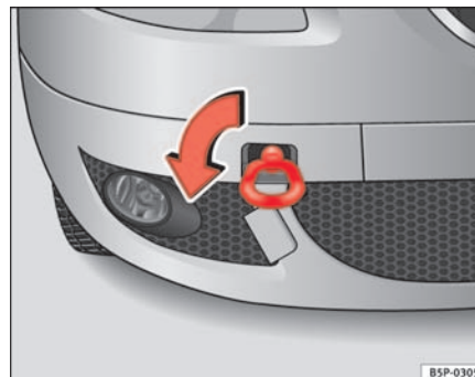
Fig. 199 Atornillado de la argolla de remolque en la parte delantera derecha del vehículo
