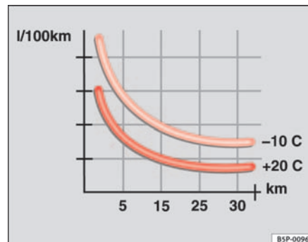
Fig. 154 Consumo de combustible (l/100 km) a dos temperaturas ambiente
