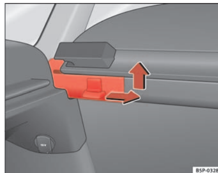
Fig. 121 Desmontaje de la bandeja portaobjetos
