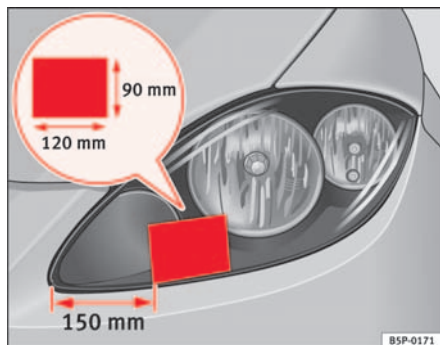
Fig. 151 Faro izquierdo
