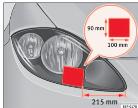
Fig. 148 Faro derecho
