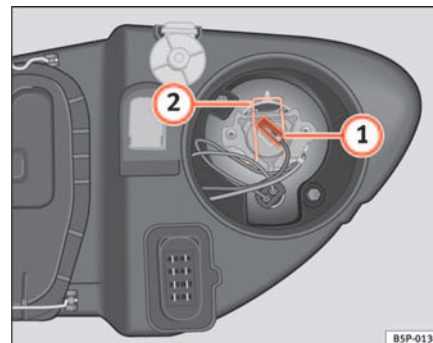
Fig. 184 Luz de carretera
