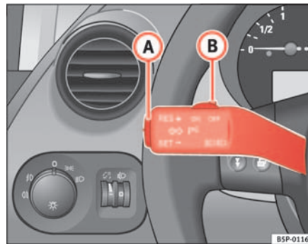
Fig. 145 Palanca de intermitentes y de luz de carretera: mando y tecla basculante para el regulador de velocidad
