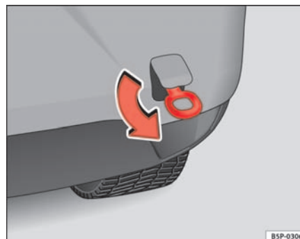
Fig. 200 Atornillado de la argolla de remolque en la parte trasera del vehículo
