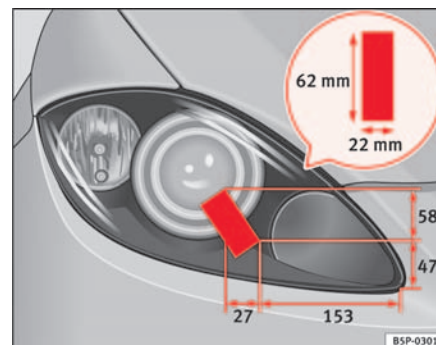
Fig. 152 Faro derecho
