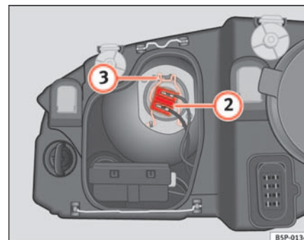
Fig. 182 Luz de cruce
