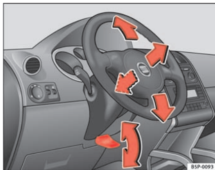
Fig. 128 Ajuste de la posición del volante
