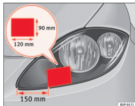
Fig. 149 Faro izquierdo
