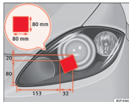
Fig. 153 Faro izquierdo ►
