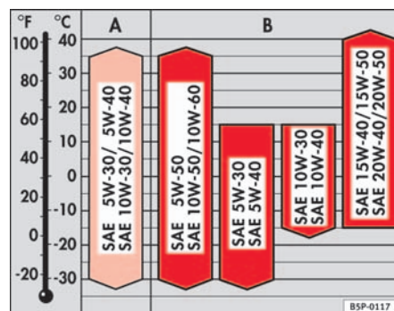
Fig. 159 Tipos de aceite de acuerdo a la temperatura
