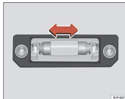
Fig. 195 Luz matrícula
