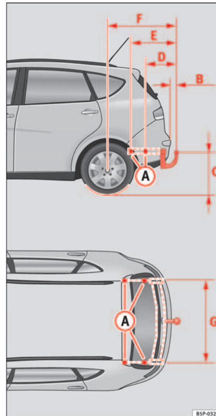
Fig. 155 Puntos de fijación del dispositivo de remolque
