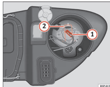
Fig. 187 Luz de carretera
