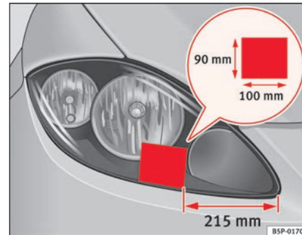
Fig. 152 Faro derecho
