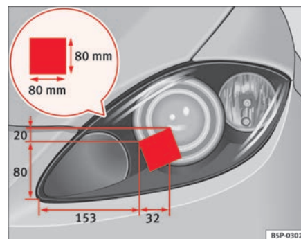
Fig. 155 Faro izquierdo
