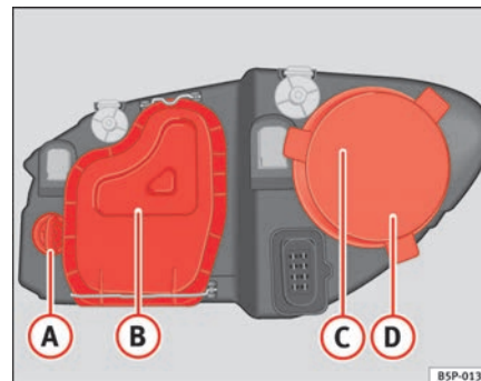
Fig. 182 Lámparas del faro principal
