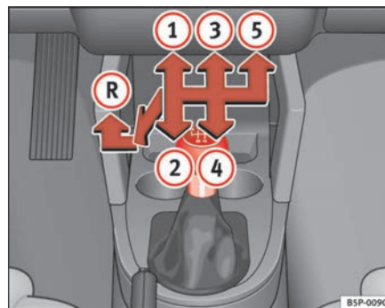
Fig. 136 Detalle de la consola central: esquema de un cambio manual de 5 marchas
