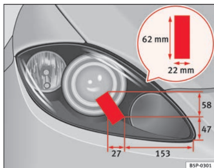
Fig. 154 Faro derecho
