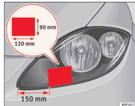
Fig. 153 Faro izquierdo ►
