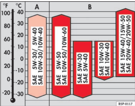
Fig. 162 Tipos de aceite de acuerdo a la temperatura
