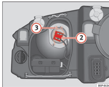
Fig. 185 Luz de cruce
