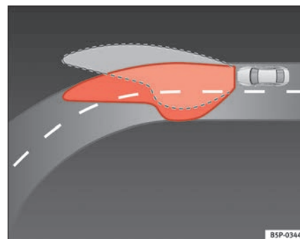
Fig. 76 Iluminación de la curva con faros autodireccionables
