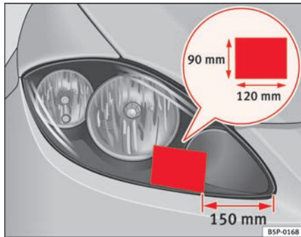
Fig. 150 Faro derecho
