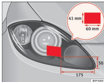
Fig. 156 Faro derecho
