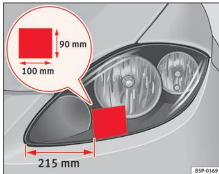
Fig. 151 Faro izquierdo
