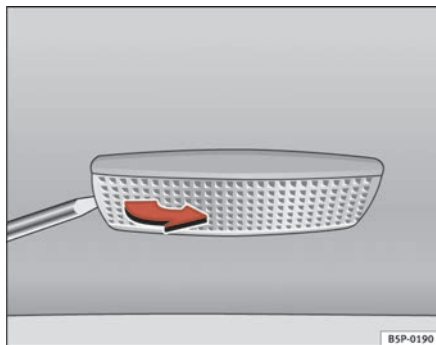
Fig. 200 Desmontaje luz del parasol
