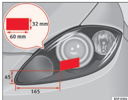
Fig. 157 Faro izquierdo
