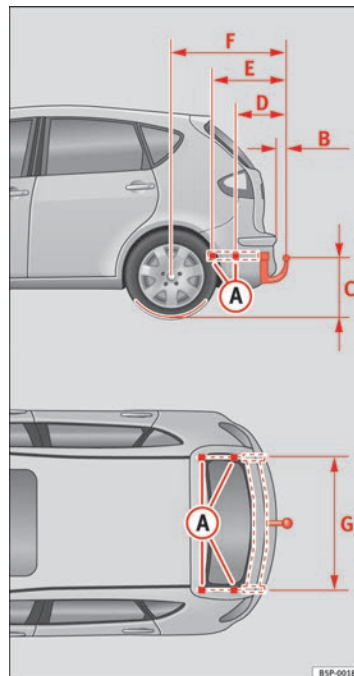
Fig. 156 Puntos de fijación del dispositivo de remolque
