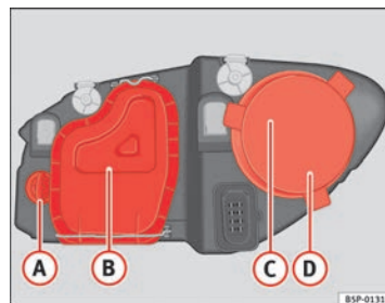
Fig. 184 Lámparas del faro principal
