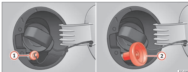
Fig. 158 Tapa del depósito abierta con boca de carga de GLP y adaptador.
