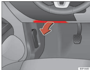
Fig. 182 Tapa de la caja de fusibles en el lado izquierdo del tablero de instrumentos
