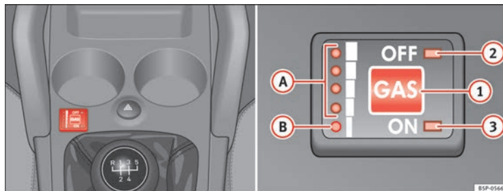
Fig. 36 Consola central: conmutador y testigos de control del sistema de gas.
