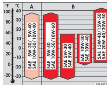
Fig. 163 Tipos de aceite de acuerdo a la temperatura
