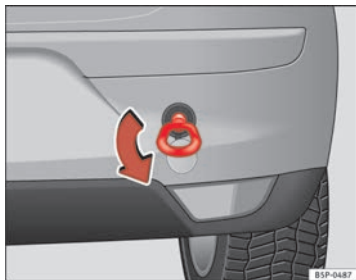
Fig. 206 Atornillado de la argolla de remolque en la parte trasera del vehículo
