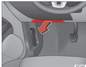
Fig. 184 Tapa de la caja de fusibles en el lado izquierdo del tablero de instrumentos
