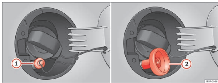
Fig. 161 Tapa del depósito abierta con boca de carga de GLP y adaptador.
