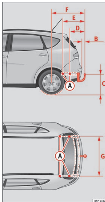
Fig. 159 Puntos de fijación del dispositivo de remolque
