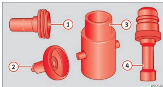
Fig. 163 Cuadro general de los adaptadores para la boca de carga de GLP.
