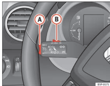
Fig. 156 Palanca de intermitentes y de luz de carretera: mando y tecla basculante para el regulador de velocidad
