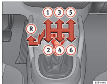
Fig. 144 Detalle de la consola central: esquema de un cambio manual de 6 marchas
