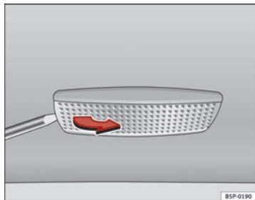
Fig. 203 Desmontaje luz del parasol
