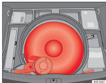
Fig. 162 Depósito de GLP en la cavidad de la rueda de repuesto.
