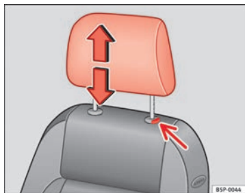
Fig. 94 Ajuste o desmontaje del apoyacabezas
