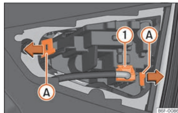
Fig. 110 Desmontar el portalámparas.
