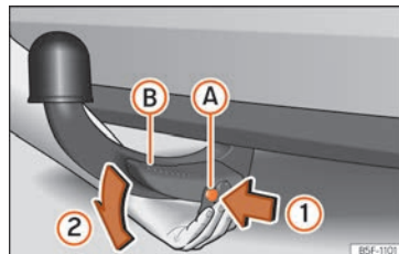
Fig. 273 Soltar la bola desmontable
