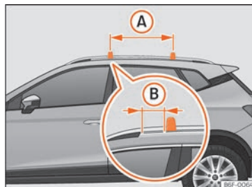
Fig. 167 Puntos de fijación de las barras longitudinales para el portaequipajes del techo.
