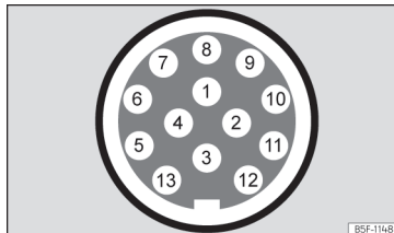
Fig. 274 Representación esquemática: asignación de los pines de la toma de corriente del remolque.
