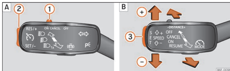
Fig. 50 A la izquierda de la columna de la dirección: A mando y teclas para manejar el regulador de velocidad; B tercera palanca para manejar el regulador de velocidad.
