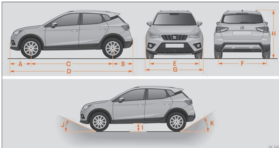
Fig. 289 Dimensiones y ángulos.
