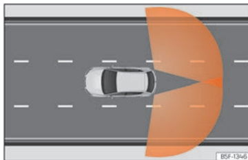
Fig. 143 Zonas de detección de los sensores
