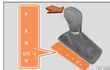
Fig. 134 Bloqueo de la palanca selectora.
