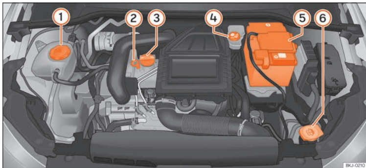
Fig. 191 Figura orientativa de la posición de los elementos.
