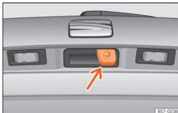
Fig. 144 En la manecilla del portón trasero: ubicación de la cámara del asistente para marcha atrás.
