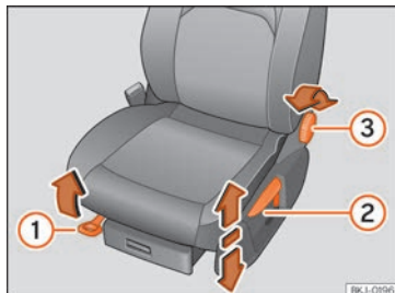
Fig. 103 Asientos delanteros: ajuste manual del asiento.
