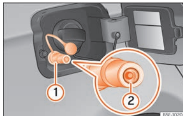
Fig. 187 Tapa del depósito abierta: boca de carga de gas ①, retén de la boca de carga ②.
