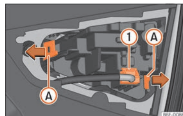
Fig. 54 Desmontar el portalámparas.
