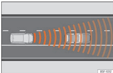
Fig. 140 Zona de detección.
