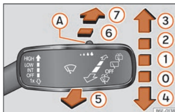
Fig. 98 Manejo del limpiaparabrisas y limpialuneta.
