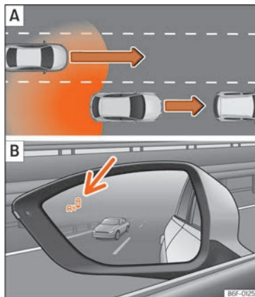
Fig. 159 Representación esquemática: A Situación en un adelantamiento con tráfico en la parte trasera. B Indicación del asistente de cambio de carril en el retrovisor exterior izquierdo.
