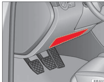
Fig. 21 Airbag de rodilla del conductor
