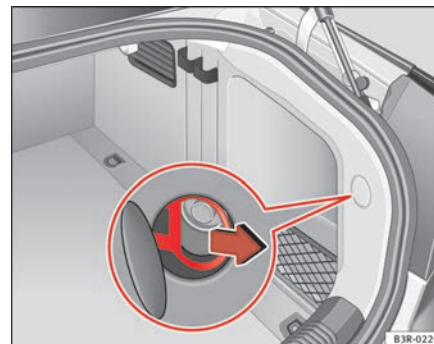
Fig. 161 Maletero: Desbloquear la tapa del depósito en caso de emergencia
