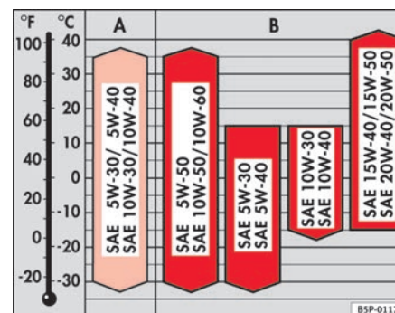
Fig. 164 Tipos de aceite de acuerdo a la temperatura
