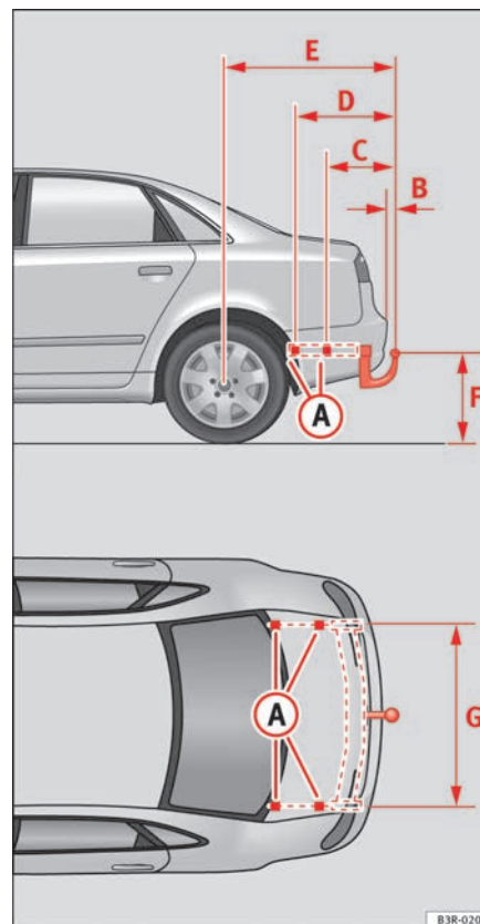
Fig. 158 Puntos de fijación del dispositivo de remolque
