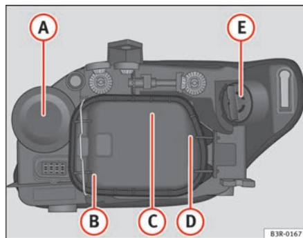
Fig. 189 Lámparas del halógeno
