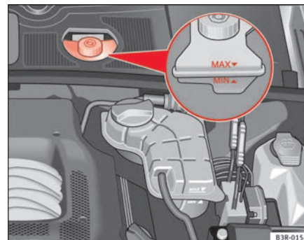
Fig. 171 Compartimento del motor: marcas en el depósito del líquido de frenos
