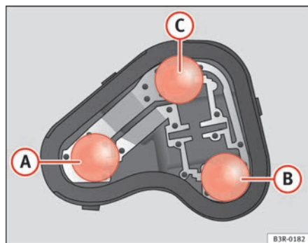
Fig. 211 Ubicación de las lámparas de incandescencia en el portalámparas: Ejemplo: Faro posterior izquierdo en la aleta.
