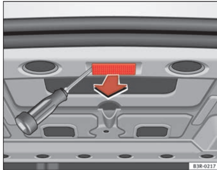
Fig. 219 Luz maletero
