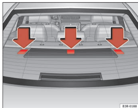
Fig. 34 Posición de las tres anillas Top Tether en la bandeja posterior
