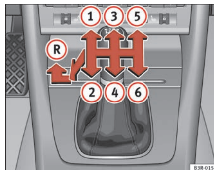
Fig. 145 Detalle de la consola central: esquema de un cambio manual de 6 marchas
