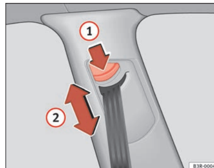
Fig. 16 Ajuste de la altura del cinturón (dispositivo-guía)
