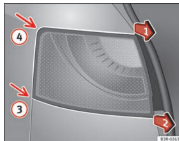
Fig. 221 Desmontar la unidad de luz trasera en la aleta
