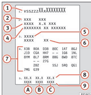
Fig. 243 Portadatos del vehículo (maletero)
