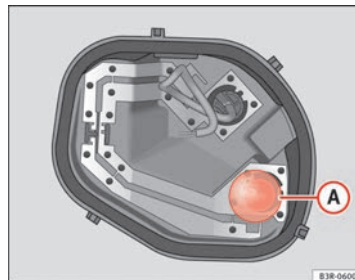
Fig. 224 Ubicación de las lámparas de incandescencia en el portalámparas: Ejemplo: Unidad de luz trasera izquierda exterior.
