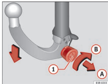
Fig. 170 Dispositivo desmontable para remolque: Desmontar la rótula
