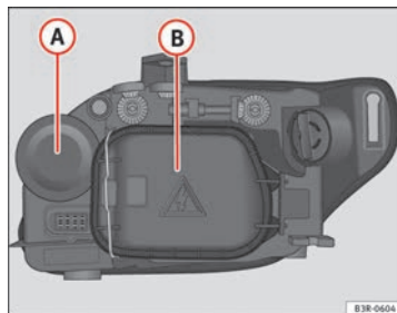
Fig. 215 Lámparas del faro Bi-Xenón AFS
