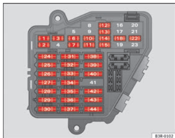
Fig. 200 Ilustración básica del portafusibles en la cubierta delantera izquierda del tablero de instrumentos: Fusibles (sin la tapa de los fusibles)
