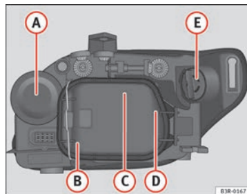
Fig. 203 Lámparas del halógeno
