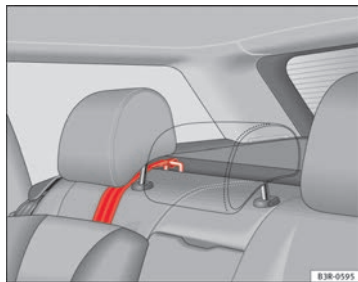
Fig. 35 Correa de sujeción: correcto ajuste y montaje
