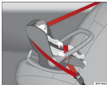
Fig. 29 Asiento para niños del grupo 0 en el asiento trasero, colocado en el sentido contrario a la dirección de la marcha.
