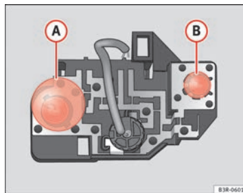
Fig. 233 Ubicación de las lámparas de incandescencia en el portalámparas. Ejemplo: Luces posteriores en el portón del maletero
