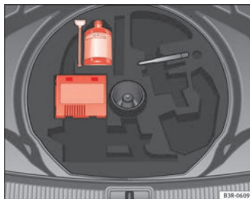
Fig. 191 Juego para reparación de neumáticos (tire mobility system) debajo de la superficie de carga del maletero
