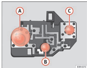
Fig. 232 Ubicación de las lámparas de incandescencia en el portalámparas. Ejemplo: Luces posteriores en el portón del maletero
