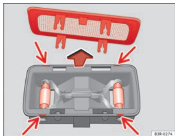
Fig. 236 Luz maletero
