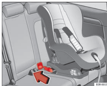
Fig. 33 Los anclajes ISOFIX del asiento infantil se deslizan por las guías de plástico ya montadas hasta fijarlos en los anclajes ISOFIX del vehículo
