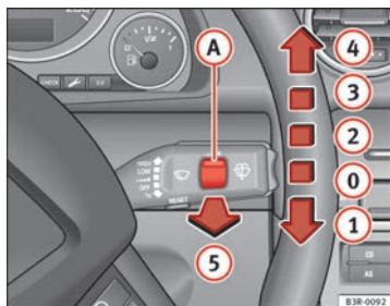
Fig. 101 Palanca del limpiaparabrisas
