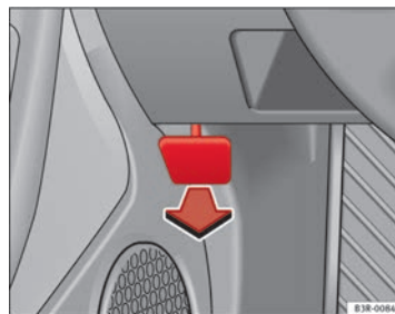
Fig. 178 Detalle de la zona reposapiés del lado del conductor: palanca para el desbloqueo del capó del motor.
