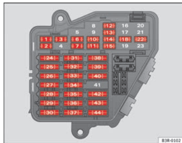
Fig. 203 Ilustración básica del portafusibles en la cubierta delantera izquierda del tablero de instrumentos: Fusibles (sin la tapa de los fusibles)
