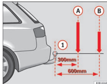
Fig. 164 Representación básica de la distribución de la carga de piezas accesorias y accesorios
