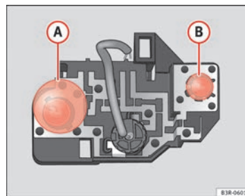
Fig. 236 Ubicación de las lámparas de incandescencia en el portalámparas. Ejemplo: Luces posteriores en el portón del maletero
