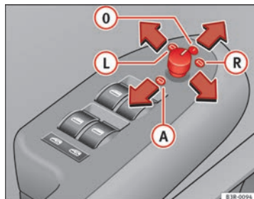
Fig. 103 Detalle del reposabrazos: Mando giratorio
