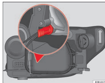
Fig. 215 Luz de posición. Empuñadura del portalámparas en posición vertical
