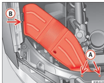
Fig. 205 Conducción de ventilación en el lado derecho del vehículo
