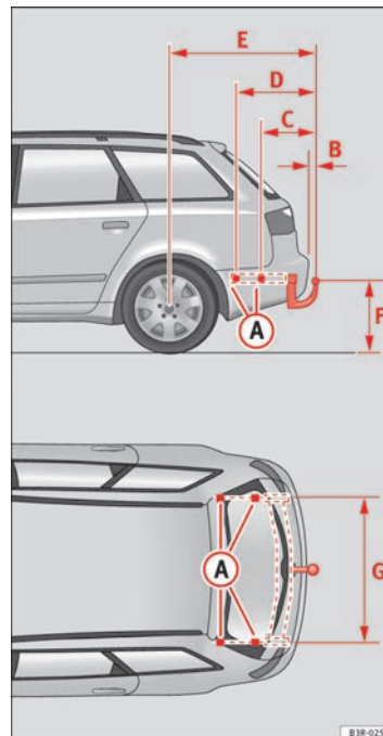
Fig. 175 Puntos de fijación del dispositivo de remolque
