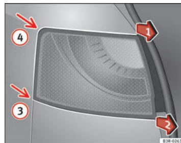
Fig. 224 Desmontar la unidad de luz trasera en la aleta
