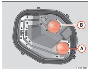
Fig. 226 Ubicación de las lámparas de incandescencia en el portalámparas: Ejemplo: Unidad de luz trasera izquierda exterior.
