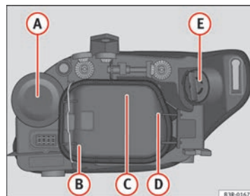
Fig. 206 Lámparas del halógeno
