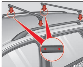
Fig. 128 Puntos de fijación de los soportes transversales
