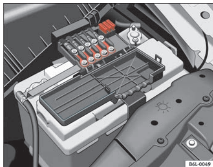
Fig. 147 Caja de fusibles sobre la batería
