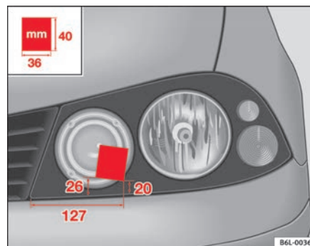
Fig. 120 Faro izquierdo
