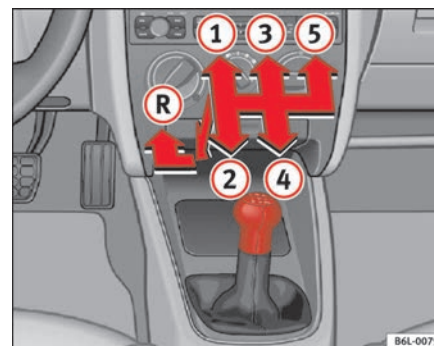
Fig. 101 Consola Central: esquema de una cambio manual de 5 marchas
