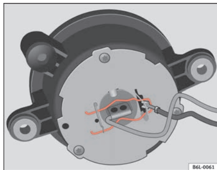
Fig. 159 Faros antiniebla
