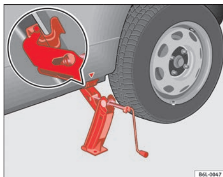
Fig. 143 Colocación del gato
