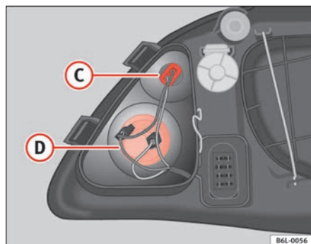
Fig. 149 Lámpara del faro principal
