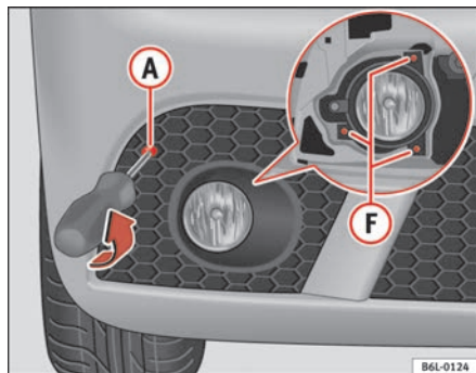
Fig. 158 Faros antiniebla
