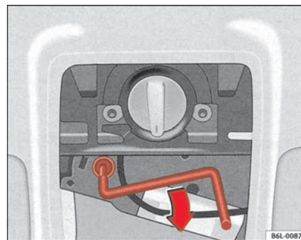
Fig. 56 Manivela cierre de emergencia
