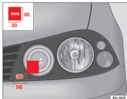
Fig. 122 Faro izquierdo
