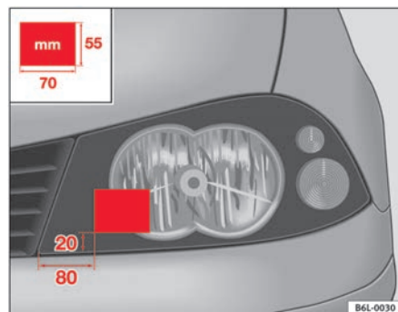
Fig. 114 Faro izquierdo
