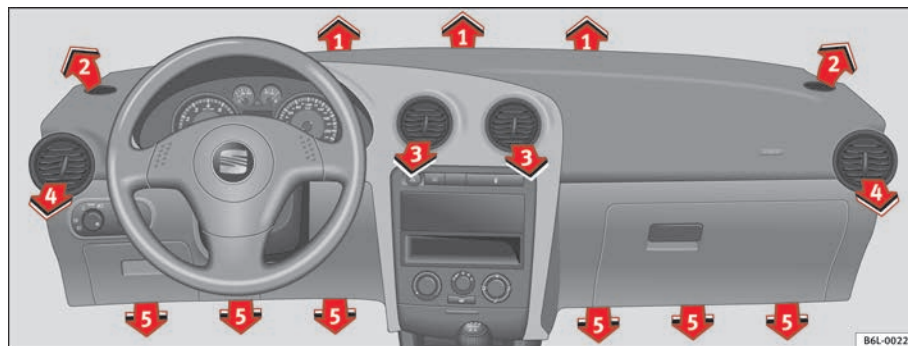
Fig. 93 Difusores de aire
