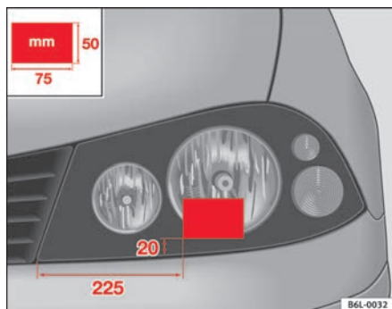
Fig. 116 Faro izquierdo
