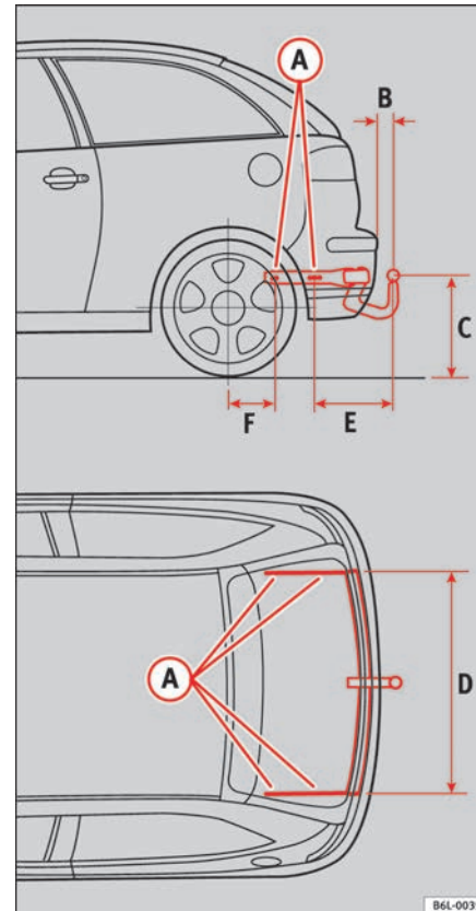
Fig. 123 Puntos de fijación del dispositivo de remolque
