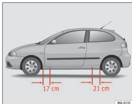
Fig. 142 Puntos de apoyo del gato
