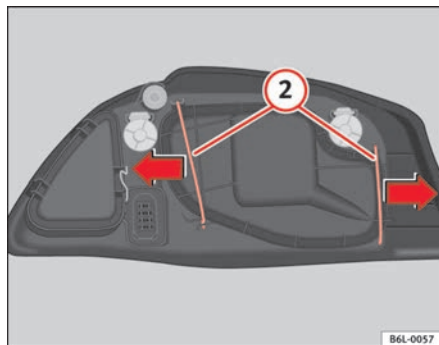
Fig. 150 Lámpara luz de cruce
