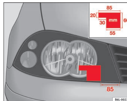
Fig. 111 Faro derecho
