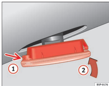
Fig. 160 Intermitentes laterales
