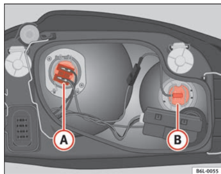
Fig. 148 Lámpara del faro principal
