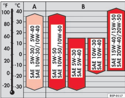
Fig. 126 Tipos de aceite de acuerdo a la temperatura
