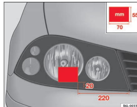
Fig. 117 Faro derecho
