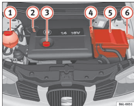
Fig. 177 Figura orientativa de la posición de los elementos
