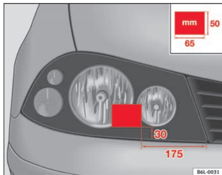
Fig. 115 Faro derecho
