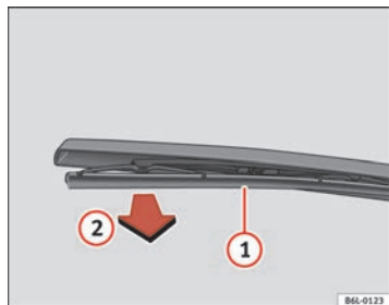
Fig. 122 Cambio de la escobilla del limpiapuneta
