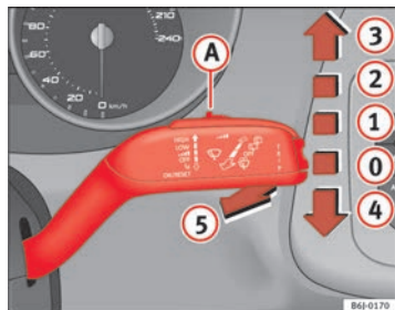
Fig. 61 Palanca del limpia-lavacristales
