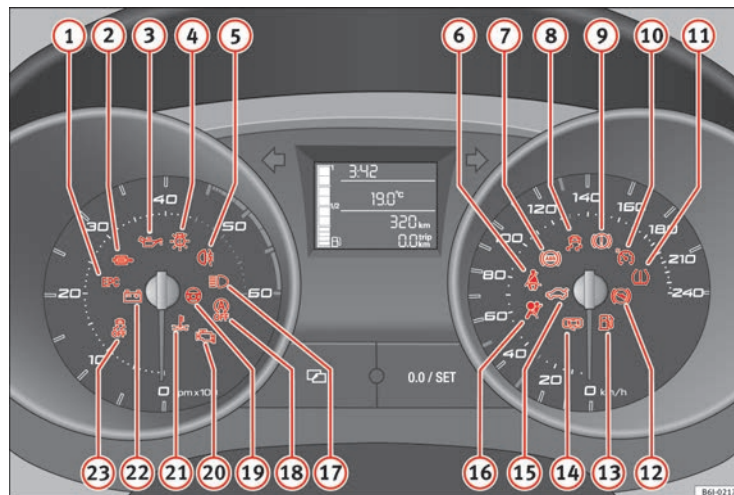
Fig. 37 Testigos de control y de advertencia del cuadro de instrumentos. Algunos de estos testigos pertenecen sólo a determinadas versiones del modelo o forman parte de equipamientos opcionales.
