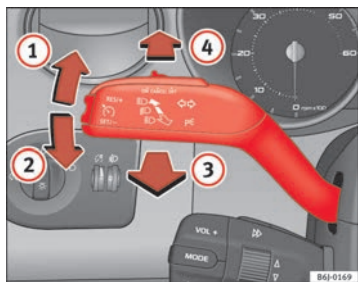
Fig. 57 Palanca de intermitentes y de luz de carretera
