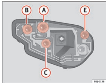
Fig. 145 Piloto izquierdo
