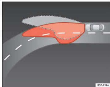
Fig. 54 Iluminación de la curva con faros autodireccionables
