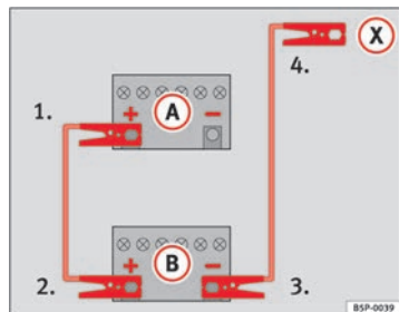
Fig. 154 Esquema para conectar los cables de emergencia en el caso de que el vehículo que suministra la corriente no disponga del sistema Start-Stop: batería descargada (A) y batería que suministra la corriente (B).
