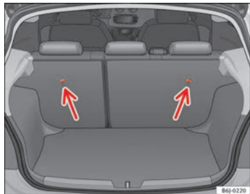
Fig. 27 Posición de las anillas Top Tether en la parte posterior del asiento trasero
