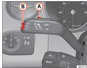
Fig. 110 Palanca de intermitentes y de luz de carretera: mando y tecla basculante para el regulador de velocidad
