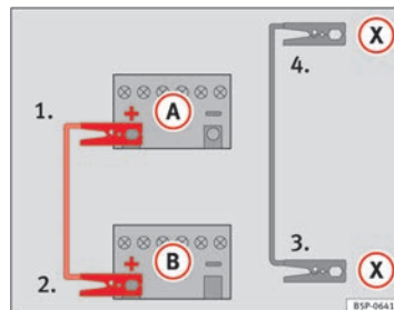
Fig. 155 Esquema para conectar los cables de emergencia en el caso de que el vehículo que suministra la corriente disponga del sistema Start-Stop: batería descargada (A) y batería que suministra la corriente (B).
