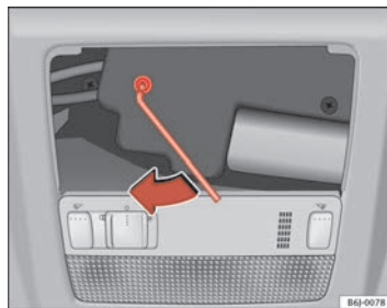
Fig. 50 Accionamiento de emergencia techo panorámico/deflector
