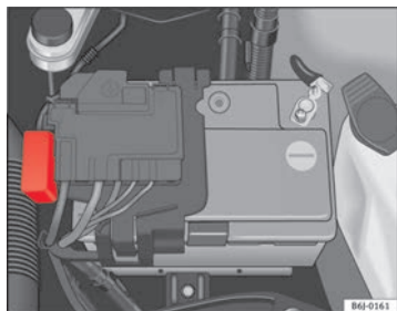
Fig. 133 Fusibles en el compartimiento motor
