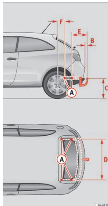
Fig. 113 Puntos de fijación del dispositivo de remolque
