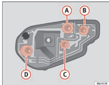
Fig. 146 Piloto derecho
