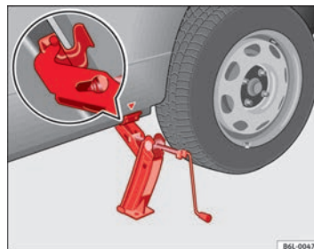
Fig. 147 Colocación del gato
