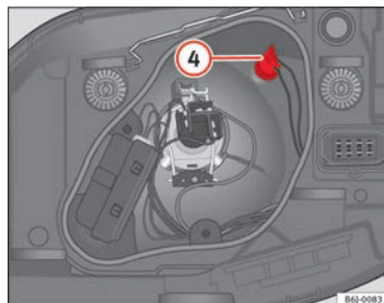
Fig. 155 Luz de posición
