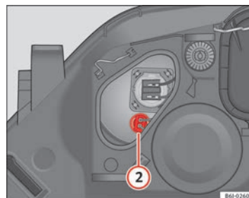
Fig. 158 Luz de posición
