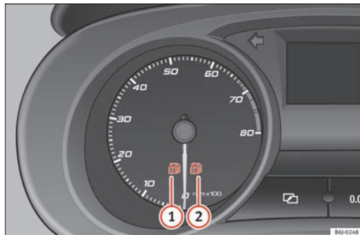
Fig. 39 Testigos de control y de advertencia del cuadro de instrumentos en vehículos con GLP.
