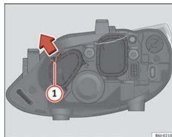
Fig. 157 Luz de posición
