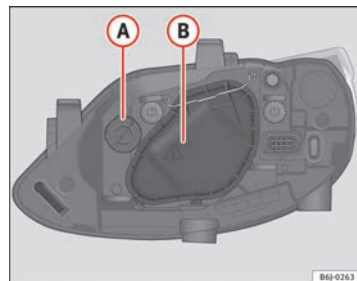
Fig. 164 Lámparas del faro AFS
