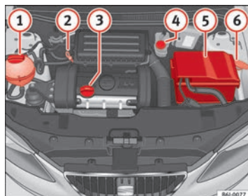
Fig. 183 Figura orientativa de la posición de los elementos
