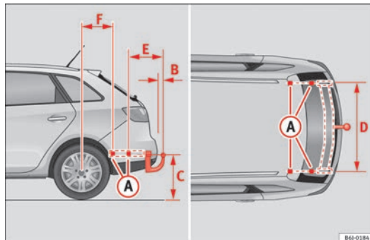
Fig. 126 Puntos de fijación del dispositivo de remolque
