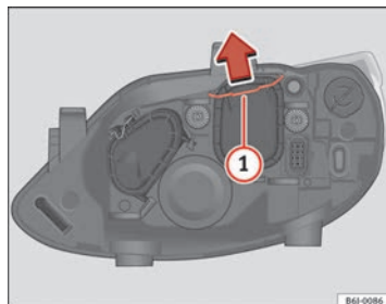
Fig. 161 Luz de cruce
