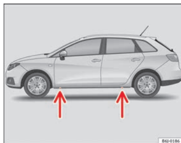
Fig. 146 Puntos de apoyo del gato
