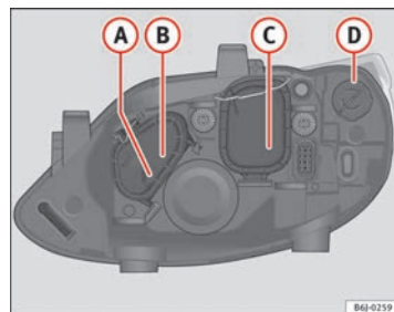
Fig. 156 Faro doble
