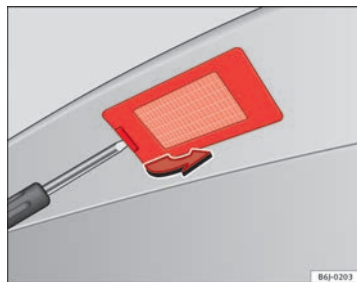
Fig. 174 Desmontaje de la luz de matrícula.
