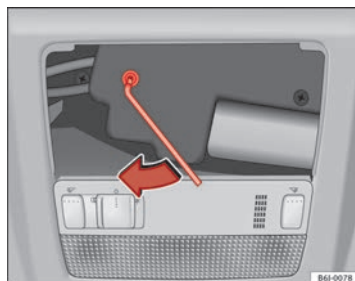
Fig. 53 Accionamiento de emergencia techo panorámico/deflector
