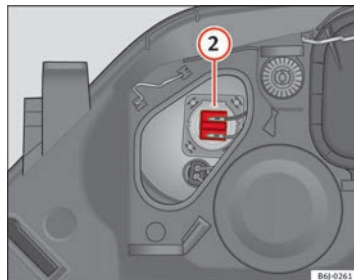
Fig. 160 Luz de carretera
