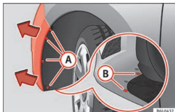
Fig. 191 Faro antiniebla: acceso al conector y al portalámparas.
