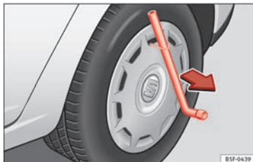
Fig. 158 Retirar el embellecedor integral.
