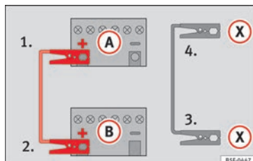
Fig. 165 Esquema de conexión para vehículos con sistema Start-Stop.
