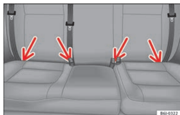
Fig. 66 Anillas de sujeción ISOFIX.
