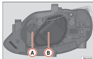
Fig. 187 Lámparas del faro AFS.
