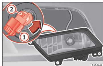
Fig. 192 Faro antiniebla.
