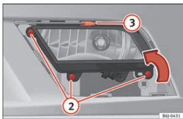
Fig. 190 Faro antiniebla.
