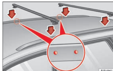
Fig. 124 Ibiza ST: puntos de fijación de las barras longitudinales para el portaequipajes del techo.
