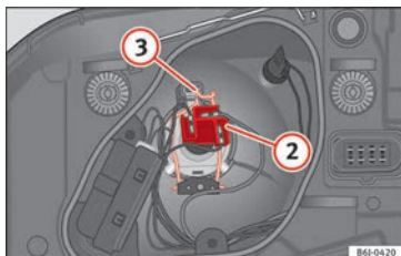
Fig. 177 Luz de cruce/carretera del faro simple.
