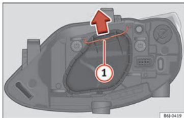
Fig. 176 Luz de cruce/carretera del faro simple.
