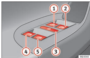
Fig. 87 Detalle de la puerta del conductor: mandos para las ventanillas delanteras y traseras (vehículo de 5 puertas con elevallas eléctricos anteriores y posteriores).
