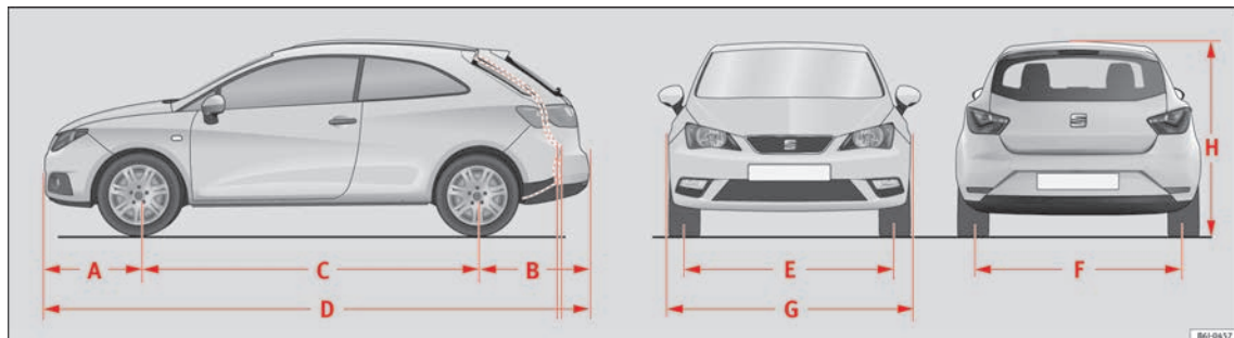
Fig. 209 Dimensiones
