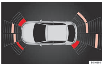
Fig. 146 Visualización de ayuda al aparcamiento en la pantalla del navegador.
