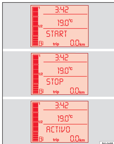
Fig. 142 Indicación en la pantalla del cuadro de instrumentos durante el funcionamiento Start-Stop.
