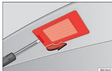
Fig. 203 Desmontaje de la luz de matrícula.
