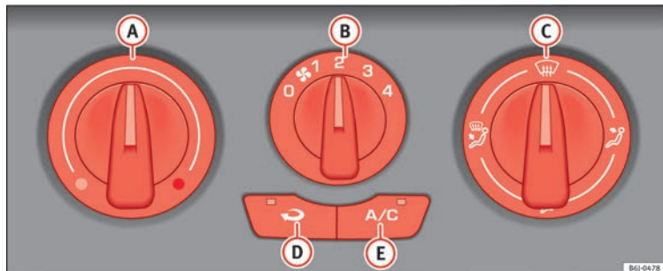
Fig. 128 Mandos del aire acondicionado en el tablero de instrumentos.
