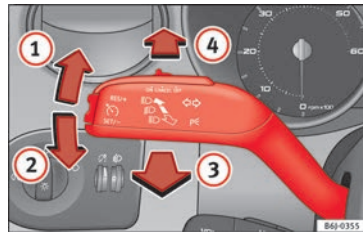
Fig. 91 Palanca de intermitentes y de luz de carretera.
