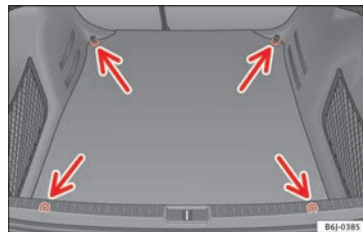
Fig. 118 Disposición de las argollas de amarre en el maletero.
