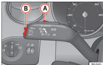
Fig. 149 Palanca de intermitentes y de luz de carretera: mando y tecla basculante para el regulador de velocidad.
