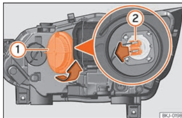
Fig. 103 En el vano motor: lámpara de luz de carretera.
