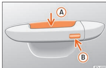
Fig. 138 Sistema de cierre y arranque sin llave Keyless Access: superficie sensora (A) de desbloqueo en la parte interior de la manecilla de la puerta y superficie sensora (B) de bloqueo en la parte exterior de la manecilla.
