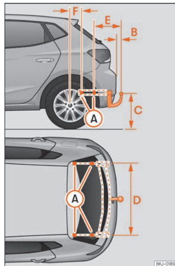
Fig. 264 Puntos de fijación del dispositivo de remolque.
