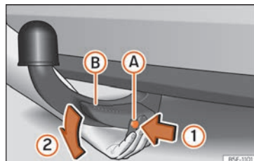
Fig. 261 Soltar la bola desmontable
