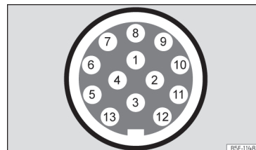
Fig. 262 Representación esquemática: asignación de los pines de la toma de corriente del remolque.
