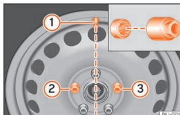
Fig. 75 Cambio de rueda: válvula del neumático (1) y lugar de montaje del tornillo de rueda antirrobo (2) o (3).
