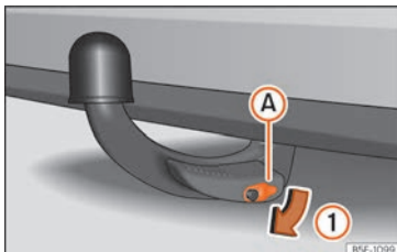
Fig. 259 Retirar la tapa de la cerradura
