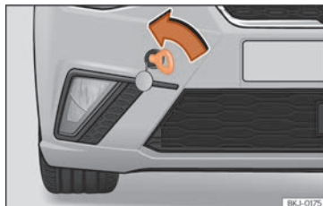
Fig. 78 Parte derecha del parachoques delantero: argolla de remolque.
