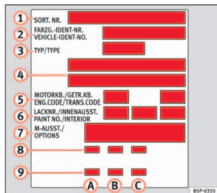
Fig. 183 Portadatos del vehículo (maletero)
