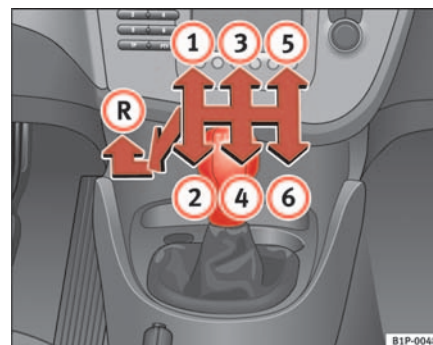
Fig. 117 Detalle de la consola central: esquema de un cambio manual de 6 marchas
