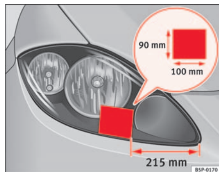
Fig. 132 Faro derecho
