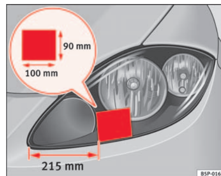
Fig. 131 Faro izquierdo
