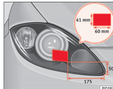
Fig. 136 Faro derecho
