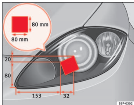
Fig. 135 Faro izquierdo
