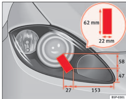
Fig. 134 Faro derecho
