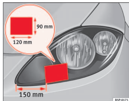
Fig. 133 Faro izquierdo
