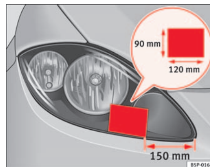
Fig. 130 Faro derecho
