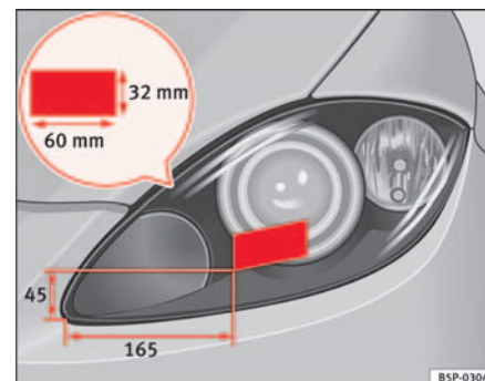
Fig. 137 Faro izquierdo ►
