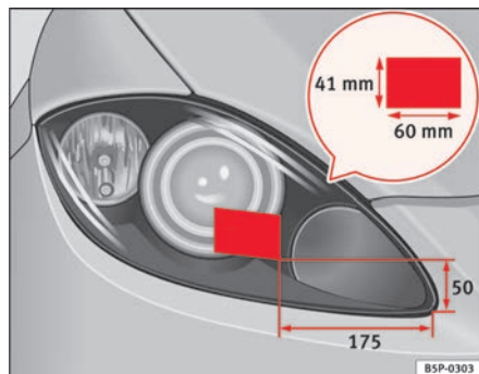
Fig. 137 Faro derecho
