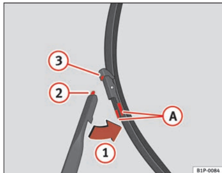
Fig. 148 Cambio de las escobillas del limpiaparabrisas
