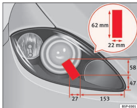
Fig. 135 Faro derecho
