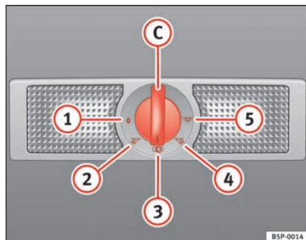
Fig. 80 Revestimiento interior del techo: iluminación interior y de lectura de la parte trasera del habitáculo.
