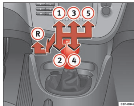
Fig. 117 Detalle de la consola central: esquema de un cambio manual de 5 marchas
