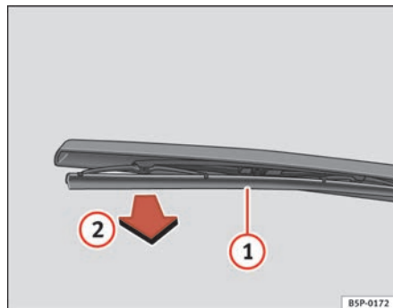
Fig. 149 Cambio de la escobilla del limpialuneta
