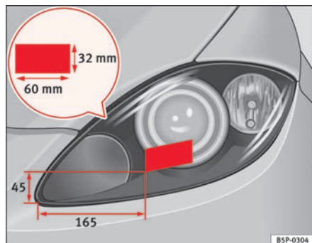
Fig. 138 Faro izquierdo
