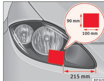
Fig. 133 Faro derecho
