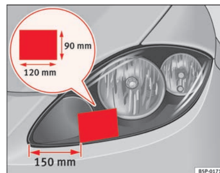
Fig. 134 Faro izquierdo ►
