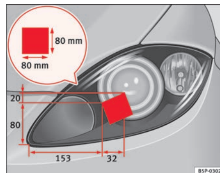
Fig. 136 Faro izquierdo
