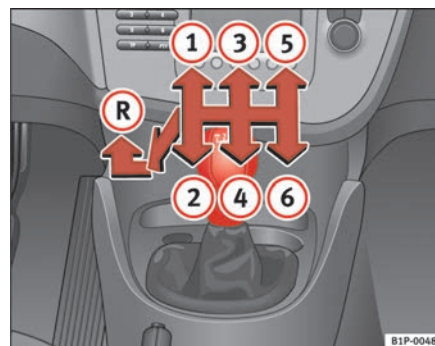
Fig. 118 Detalle de la consola central: esquema de un cambio manual de 6 marchas
