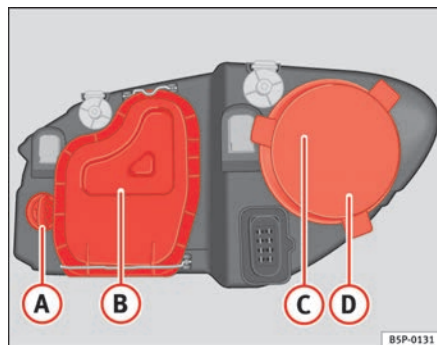
Fig. 162 Lámparas del faro principal
