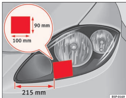
Fig. 132 Faro izquierdo
