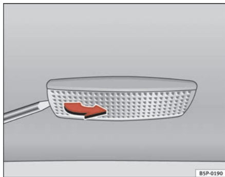
Fig. 174 Desmontaje luz del parabol
