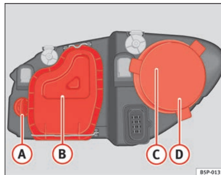
Fig. 158 Lámparas del faro principal
