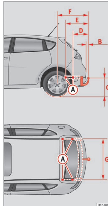
Fig. 134 Puntos de fijación del dispositivo de remolque
