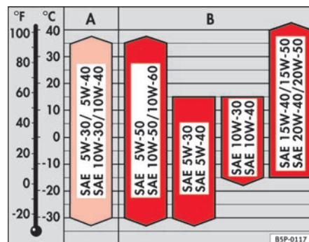
Fig. 138 Tipos de aceite de acuerdo a la temperatura
