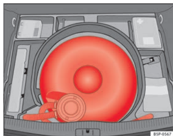
Fig. 138 Depósito de GLP en la cavidad de la rueda de repuesto.
