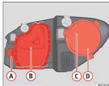
Fig. 162 Lámparas del faro principal
