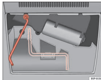
Fig. 69 Manivela cierre de emergencia
