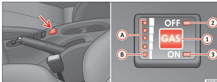
Fig. 35 Consola central: conmutador y testigos de control del sistema de gas.
