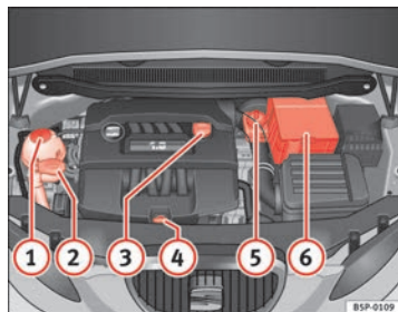
Fig. 184 Figura orientativa de la posición de los elementos
