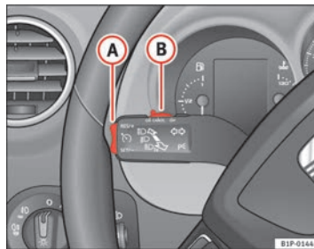
Fig. 134 Palanca de intermitentes y de luz de carretera: mando y tecla basculante para el regulador de velocidad
