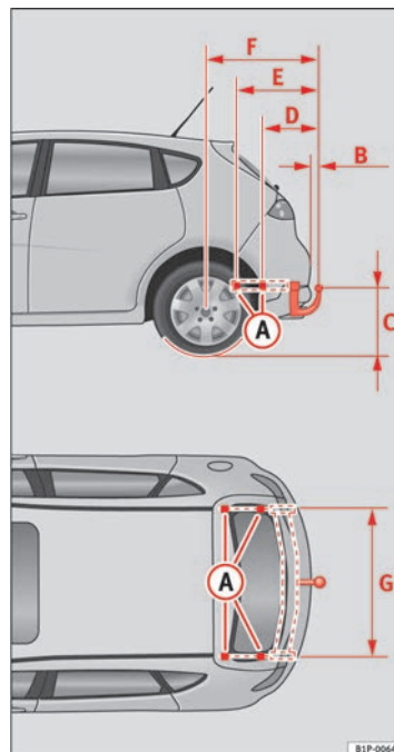
Fig. 135 Puntos de fijación del dispositivo de remolque
