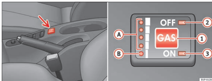
Fig. 117 Consola central: conmutador y testigos de control del sistema de gas.
