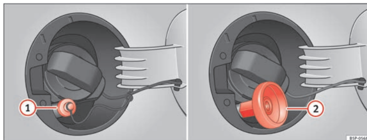
Fig. 137 Tapa del depósito abierta con boca de carga de GLP y adaptador.
