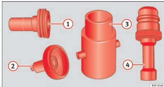
Fig. 139 Cuadro general de los adaptadores para la boca de carga de GLP.
