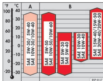
Fig. 142 Tipos de aceite de acuerdo a la temperatura
