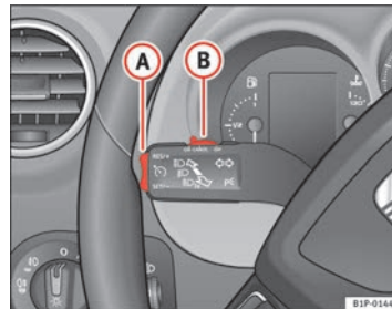
Fig. 133 Palanca de intermitentes y de luz de carretera: mando y tecla basculante para el regulador de velocidad
