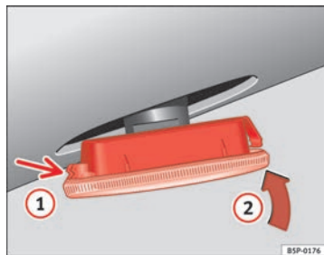
Fig. 173 Intermitente lateral
