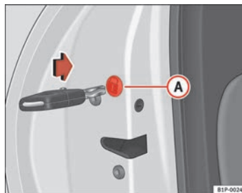
Fig. 57 Cierre de emergencia de las puertas
