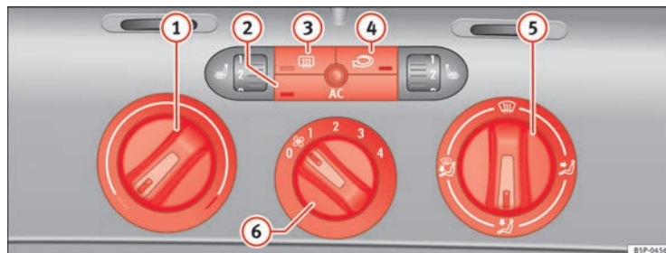
Fig. 108 Mandos del Climatic en el tablero de instrumentos
