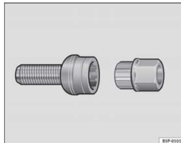
Fig. 121 Tornillo antirrobo de la rueda con capuchón y adaptador
