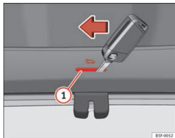
Fig. 55 Detalle del maletero: acceso al desbloqueo de emergencia
