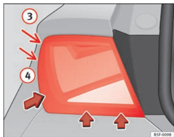
Fig. 144 Desmontar la unidad de luz trasera en la aleta
