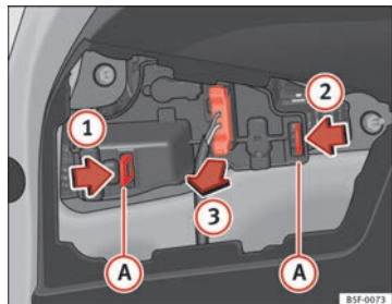
Fig. 147 Desmontar el portalámparas
