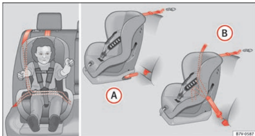
Fig. 31 En los asientos traseros: la ilustración (A) muestra la fijación básica del sistema de retención para niños con las anillas de sujeción inferiores y el cinturón de sujeción superior. La ilustración (B) muestra la fijación del sistema de retención para niños con el cinturón de seguridad del vehículo.
