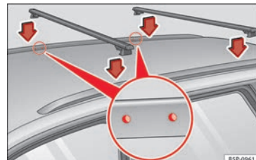
Fig. 139 Leon ST: puntos de fijación de las barras longitudinales para el portaequipajes del techo.
