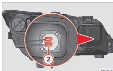
Fig. 211 Lámpara de luz de carretera.
