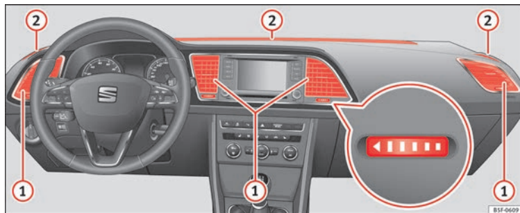
Fig. 140 En el tablero de instrumentos: difusores de aire.
