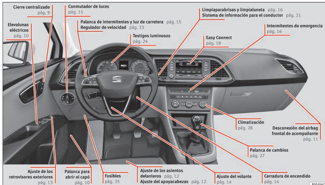
Fig. 3 Guía izquierda
