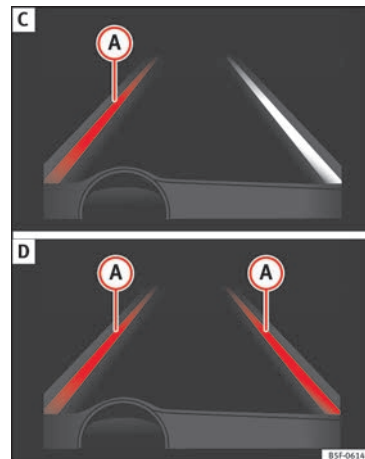
Fig. 163 En la pantalla del cuadro de instrumentos: indicación en la pantalla del sistema de aviso de salida del carril (ejemplo 2).
