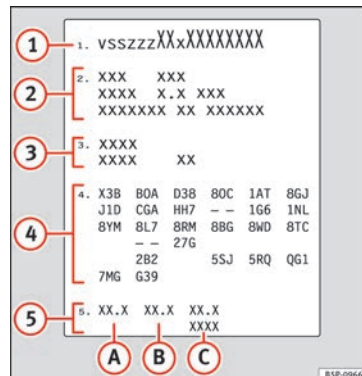
Fig. 225 Portadatos del vehículo (maletero).
