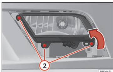
Fig. 213 Faro antiniebla.
