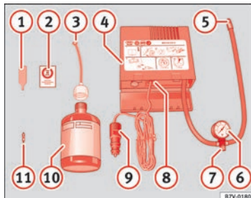
Fig. 188 Representación estándar: contenido del kit antipinchazos.
