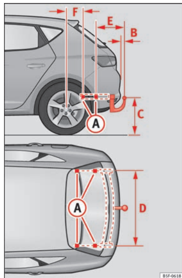
Fig. 172 Puntos de fijación del dispositivo de remolque.
