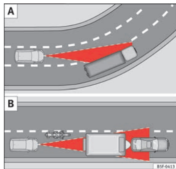
Fig. 156 (A) Vehículo en una curva. (B) Motociclista circulando por delante fuera del radio de acción del sensor de radar.
