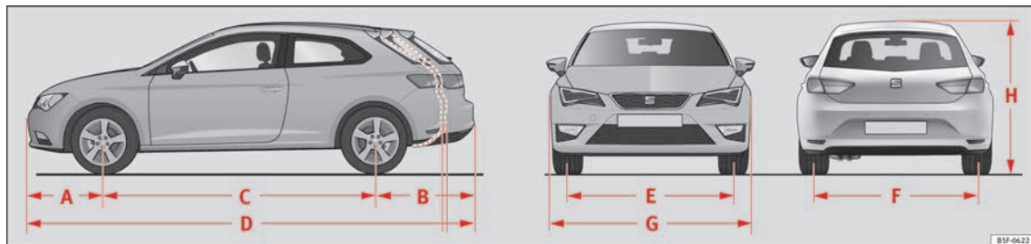
Fig. 227 Dimensiones
