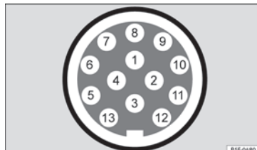
Fig. 171 Representación esquemática: asignación de los pines de la toma de corriente del remolque.
