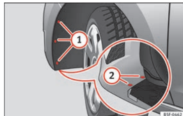
Fig. 214 Faro antiniebla: acceso al conector y al portalámparas.
