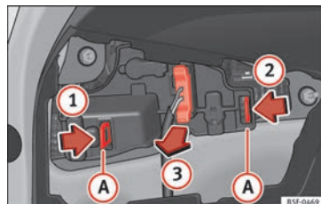
Fig. 221 Desmontar el portalámparas.
