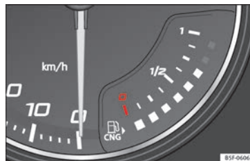
Fig. 85 Indicador de combustible.
